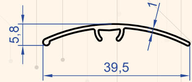
Profil No : 1008 Gramaj : 0.140 kg/m
