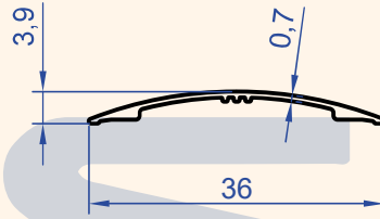
Profil No : 1001 Gramaj : 0.089 kg/m
