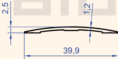
Profil No : 1060 Gramaj : 0.128 kg/m
