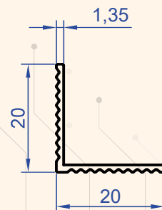
Profil No : 1017 Gramaj : 0.117 kg/m
