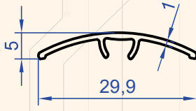
Profil No : 1018 Gramaj : 0.107 kg/m
