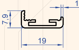
Profil No : 4053 Gramaj : 0.134 kg/m
