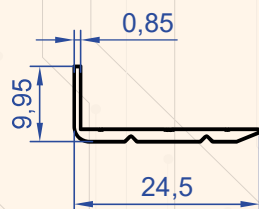
Profil No : 1185 Gramaj : 0.117 kg/m
