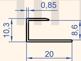
Profil No : 1050 Gramaj : 0.087 kg/m
