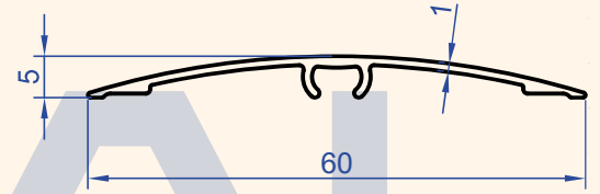
Profil No : 1019 Gramaj : 0.201 kg/m
