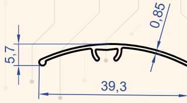
Profil No : 1014 Gramaj : 0.120 kg/m
