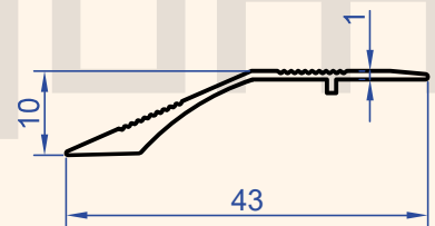
Profil No : 1049 Gramaj : 0.168 kg/m
