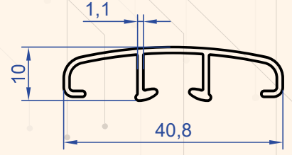
Profil No : 9207 Gramaj : 0.240 kg/m
