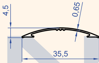
Profil No : 1054 Gramaj : 0.080 kg/m
