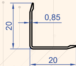
Profil No : 1009 Gramaj : 0.086 kg/m
