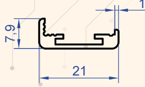
Profil No : 2659 Gramaj : 0.148 kg/m
