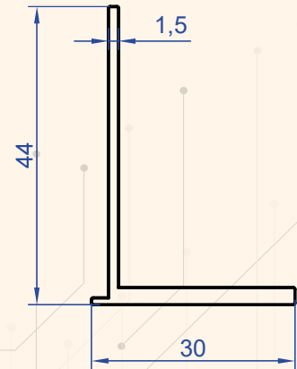
Profil No : 1326 Gramaj : 0.361 kg/m
