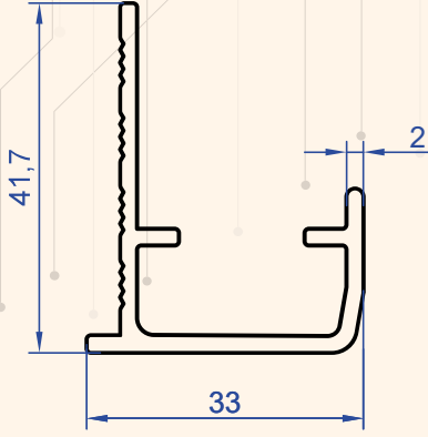
Profil No : 1372 Gramaj : 0.530 kg/m
