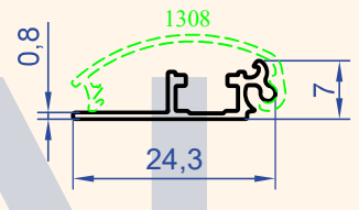
Profil No : 1310 Gramaj : 0.101 kg/m
