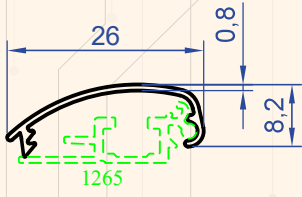
Profil No : 1265 Gramaj : 0.087 kg/m
