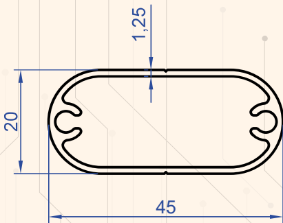
Profil No : 1263 Gramaj : 0.457 kg/m
