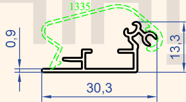
Profil No : 1335 Gramaj : 0.162 kg/m
