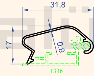
Profil No : 1336 Gramaj : 0.135 kg/m
