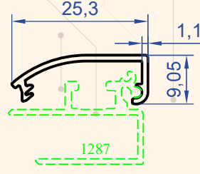
Profil No : 1287 Gramaj : 0.121 kg/m
