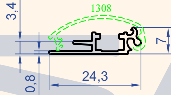
Profil No : 1308 Gramaj : 0.112 kg/m
