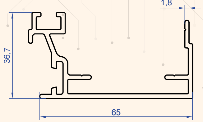
Profil No : 1373 Gramaj : 0.986 kg/m
