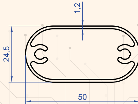
Profil No : 1390 Gramaj : 0.625 kg/m
