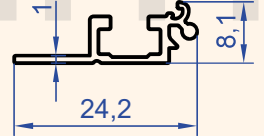
Profil No : 1345 Gramaj : 0.125 kg/m
