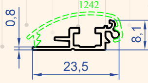
Profil No : 1242 Gramaj : 0.125 kg/m
