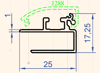
Profil No : 1288 Gramaj : 0.218 kg/m
