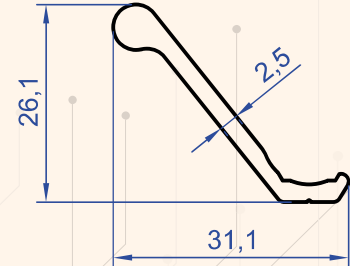
Profil No : 1168 Gramaj : 0.316 kg/m
