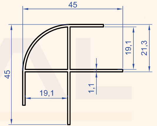
Profil No : 1924 Gramaj : 0.445 kg/m
