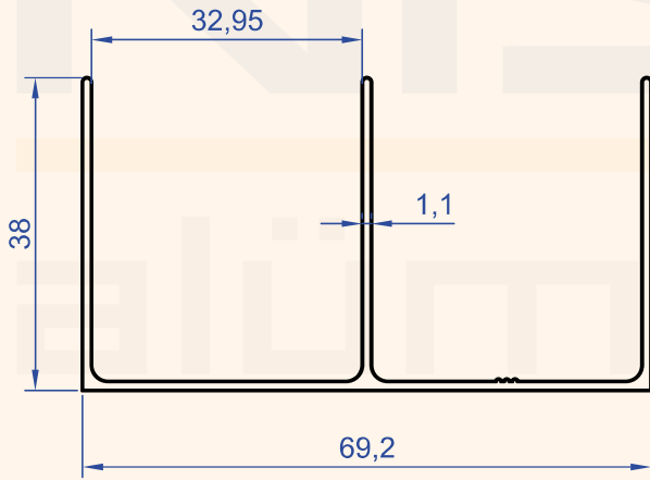
Profil No : 6307 Gramaj : 0.545 kg/m
