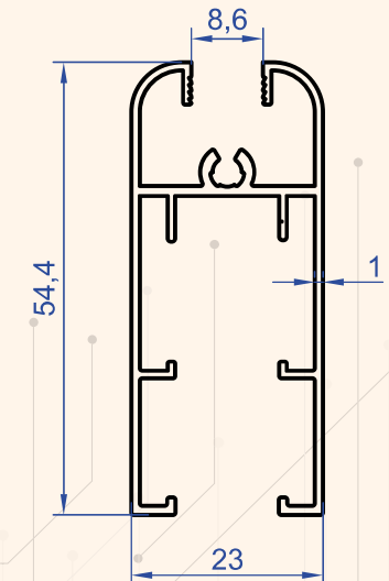
Profil No : 1316 Gramaj : 0.519 kg/m
