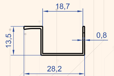
Profil No : 1067 Gramaj : 0.125 kg/m
