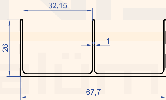
Profil No : 1045 Gramaj : 0.426 kg/m
