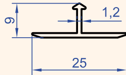
Profil No : 4641 Gramaj : 0.106 kg/m
