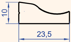
Profil No : 7163 Gramaj : 0.431 kg/m
