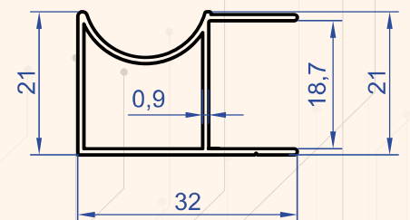
Profil No : 1388 Gramaj : 0.259 kg/m
