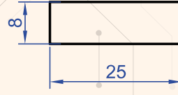
Profil No : 6 Gramaj : 0.542 kg/m
