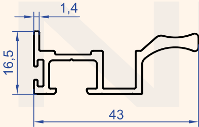
Profil No : 1238 Gramaj : 0.441 kg/m
