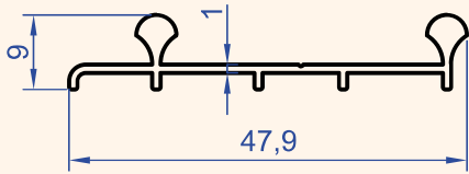
Profil No : 6823 Gramaj : 0.241 kg/m
