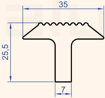
Profil No : 9559 Gramaj : 0.870 kg/m
