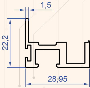
Profil No : 6918 Gramaj : 0.423 kg/m
