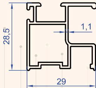
Profil No : 1175 Gramaj : 0.425 kg/m
