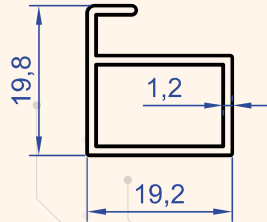
Profil No : 2670 Gramaj : 0.233 kg/m
