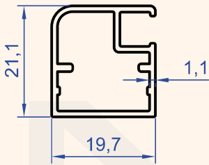
Profil No : 4497 Gramaj : 0.274 kg/m
