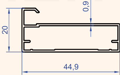
Profil No : 1131 Gramaj : 0.336 kg/m
