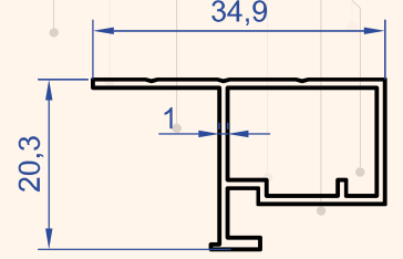
Profil No : 1191 Gramaj : 0.258 kg/m
