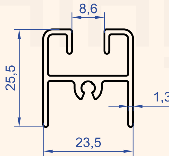
Profil No : 4622 Gramaj : 0.382 kg/m
