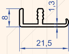
Profil No : 1923 Gramaj : 0.149 kg/m
