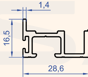
Profil No : 1239 Gramaj : 0.311 kg/m
