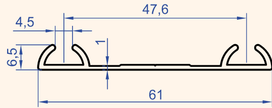
Profil No : 4831 Gramaj : 0.301 kg/m
