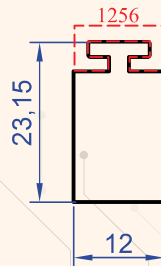
Profil No : 1257 Gramaj : 0.683 kg/m
