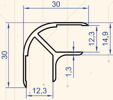
Profil No : 1201 Gramaj : 0.365 kg/m
