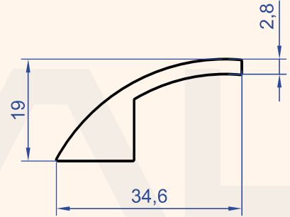
Profil No : 7161 Gramaj : 0.509 kg/m
