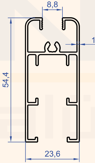
Profil No : 6750 Gramaj : 0.545 kg/m
