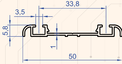
Profil No : 7498 Gramaj : 0.230 kg/m
