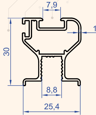
Profil No : 6301 Gramaj : 0.379 kg/m
