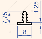
Profil No : 6932 Gramaj : 0.065 kg/m
