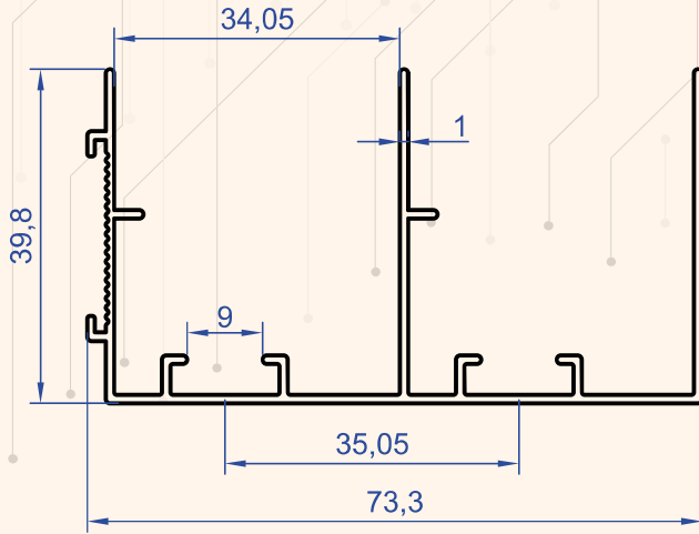
Profil No : 1212 Gramaj : 0.608 kg/m
