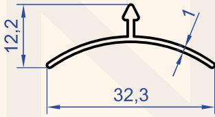
Profil No : 1324 Gramaj : 0.119 kg/m
