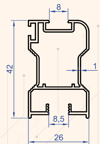
Profil No : 6816 Gramaj : 0.477 kg/m
