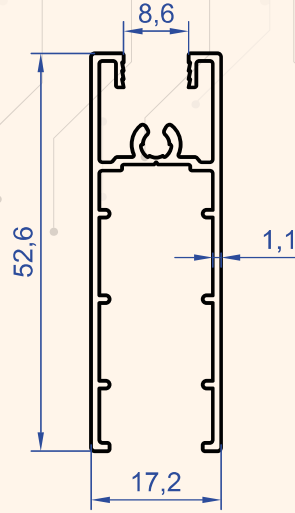
Profil No : 7522 Gramaj : 0.455 kg/m
