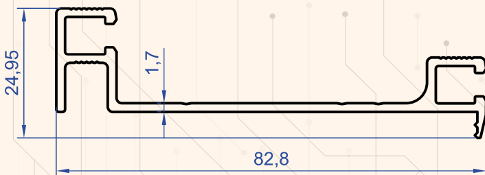
Profil No : 1187 Gramaj : 0.674 kg/m
