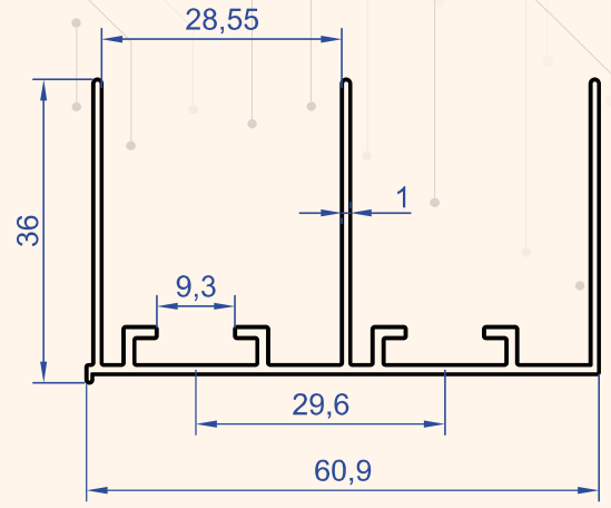
Profil No : 7429 Gramaj : 0.558 kg/m
