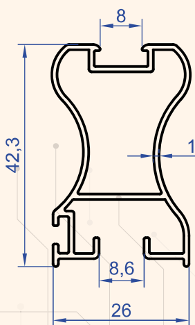
Profil No : 6415 Gramaj : 0.453 kg/m
