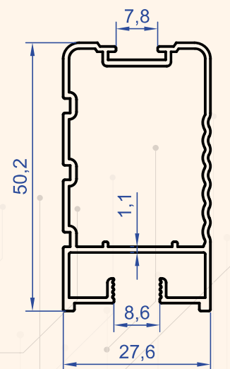
Profil No : 4945 Gramaj : 0.558 kg/m
