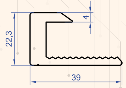
Profil No : 1347 Gramaj : 0.774 kg/m
