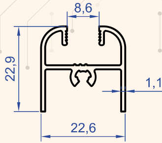
Profil No : 6353 Gramaj : 0.287 kg/m
