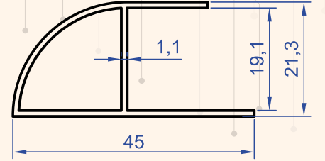
Profil No : 1926 Gramaj : 0.330 kg/m
