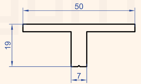
Profil No : 1255 Gramaj : 0.755 kg/m
