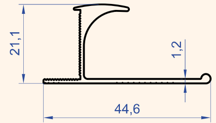
Profil No : 1244 Gramaj : 0.305 kg/m
