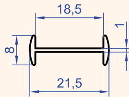
Profil No : 1048 Gramaj : 0.105 kg/m
