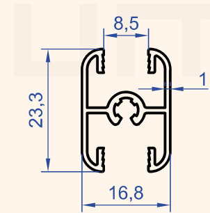
Profil No : 4946 Gramaj : 0.260 kg/m
