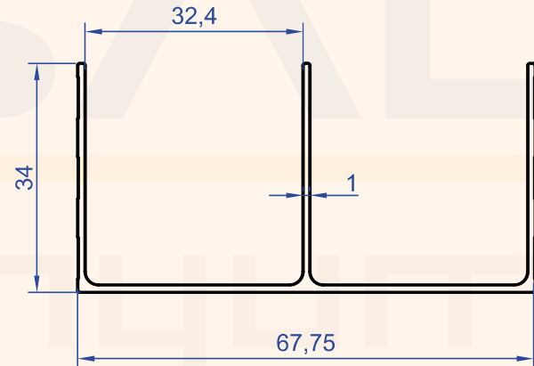
Profil No : 1276 Gramaj : 0.486 kg/m
