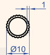
Profil No : 1026 Gramaj : 0.065 kg/m
