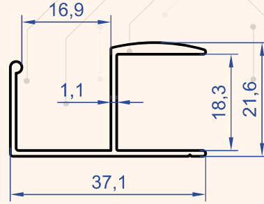
Profil No : 6705 Gramaj : 0.306 kg/m
