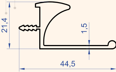
Profil No : 4427 Gramaj : 0.519 kg/m
