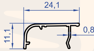
Profil No : 1292 Gramaj : 0.117 kg/m
