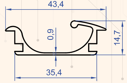
Profil No : 8642 Gramaj : 0.371 kg/m
