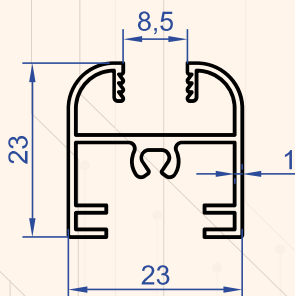
Profil No : 6874 Gramaj : 0.312 kg/m
