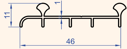
Profil No : 6819 Gramaj : 0.276 kg/m
