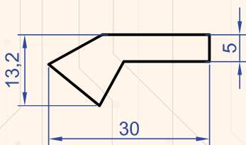
Profil No : 6293 Gramaj : 0.493 kg/m
