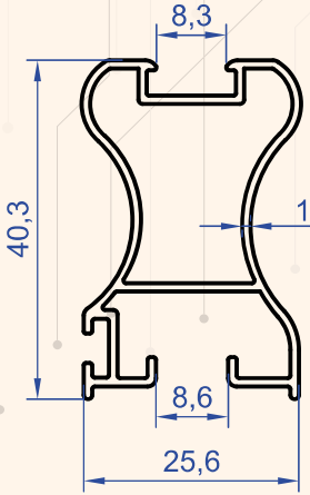
Profil No : 1135 Gramaj : 0.433 kg/m
