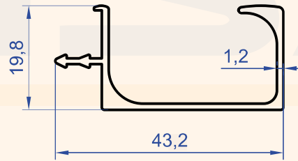
Profil No : 9056 Gramaj : 0.350 kg/m
