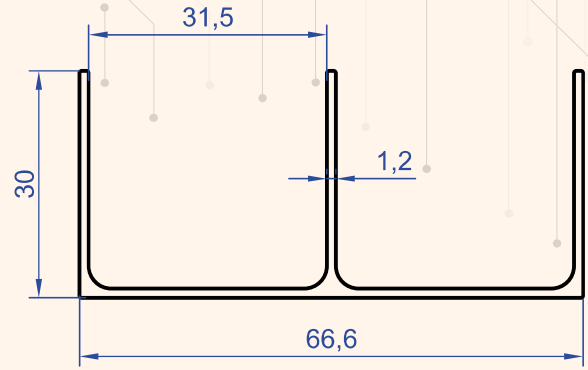
Profil No : 1913 Gramaj : 0.518 kg/m
