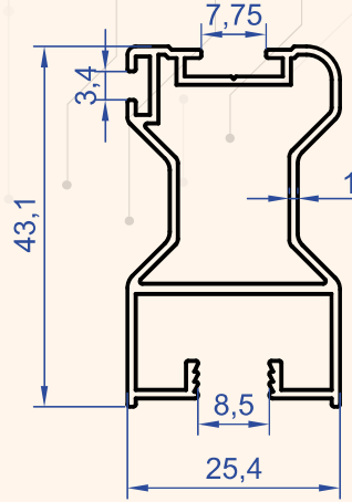
Profil No : 4839 Gramaj : 0.501 kg/m
