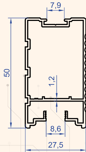
Profil No : 6441 Gramaj : 0.558 kg/m
