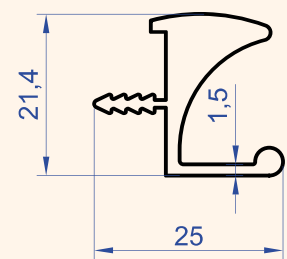
Profil No : 4426 Gramaj : 0.429 kg/m
