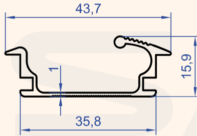
Profil No : 1370 Gramaj : 0.293 kg/m
