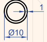
Profil No : 1022 Gramaj : 0.079 kg/m
