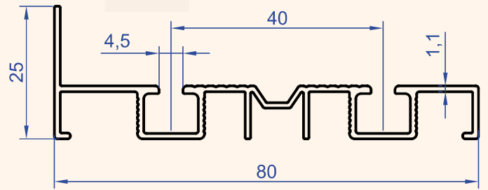
Profil No : 1186 Gramaj : 0.548 kg/m
