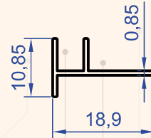
Profil No : 1034 Gramaj : 0.085 kg/m
