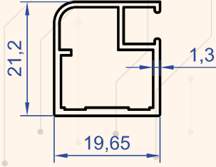
Profil No : 6849 Gramaj : 0.268 kg/m
