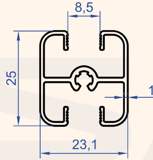
Profil No : 6756 Gramaj : 0.328 kg/m
