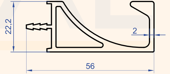
Profil No : 6184 Gramaj : 0.848 kg/m
