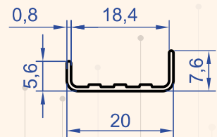
Profil No : 1012 Gramaj : 0.070 kg/m
