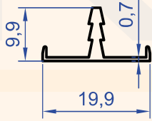
Profil No : 2889 Gramaj : 0.097 kg/m
