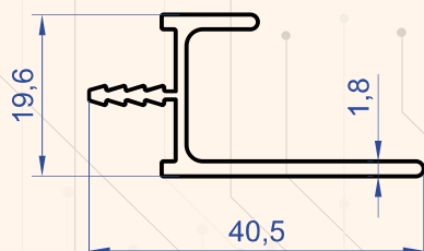
Profil No : 4562 Gramaj : 0.318 kg/m
