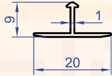
Profil No : 1024 Gramaj : 0.076 kg/m
