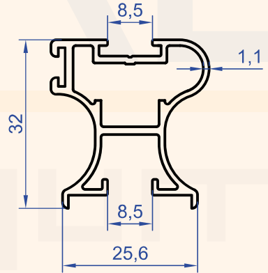
Profil No : 2698 Gramaj : 0.487 kg/m
