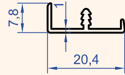
Profil No : 6109 Gramaj : 0.106 kg/m
