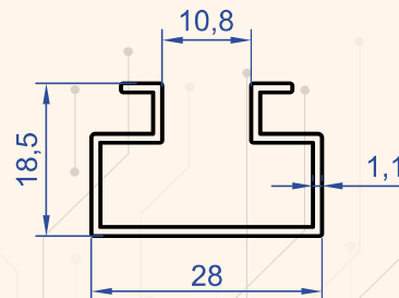
Profil No : 6111 Gramaj : 0.255 kg/m
