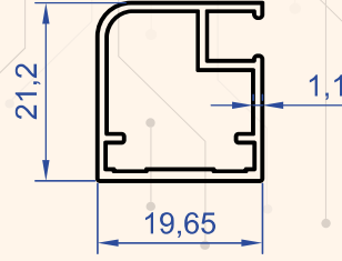
Profil No : 4310 Gramaj : 0.263 kg/m
