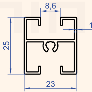
Profil No : 7502 Gramaj : 0.317 kg/m
