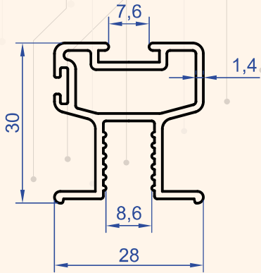
Profil No : 6626 Gramaj : 0.546 kg/m
