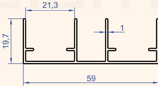
Profil No : 6724 Gramaj : 0.398 kg/m
