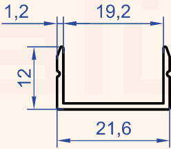
Profil No : 6846 Gramaj : 0.130 kg/m
