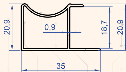
Profil No : 1103 Gramaj : 0.250 kg/m
