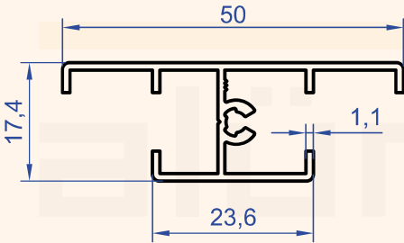
Profil No : 6901 Gramaj : 0.355 kg/m
