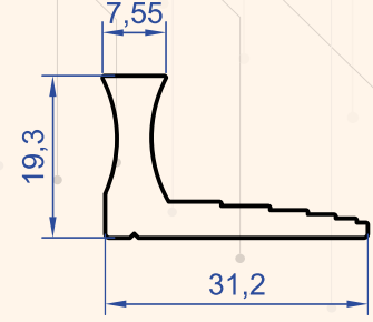
Profil No : 1108 Gramaj : 0.523 kg/m
