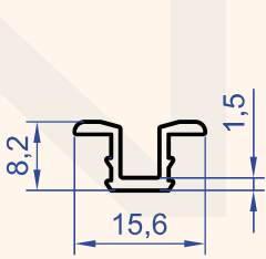
Profil No : 4635 Gramaj : 0.102 kg/m
