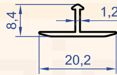
Profil No : 1133 Gramaj : 0.086 kg/m
