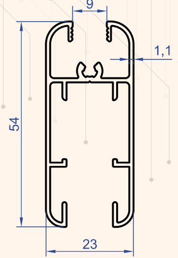
Profil No : 6721 Gramaj : 0.572 kg/m
