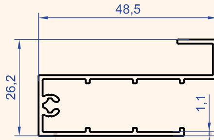
Profil No : 1174 Gramaj : 0.417 kg/m
