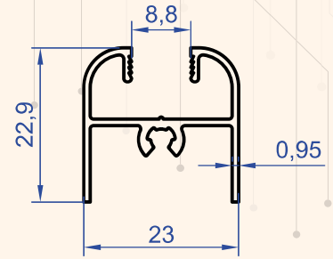
Profil No : 1315 Gramaj : 0.255 kg/m
