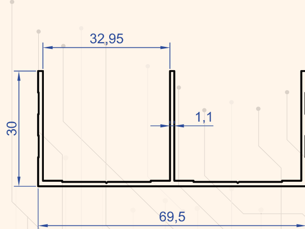
Profil No : 6782 Gramaj : 0.537 kg/m
