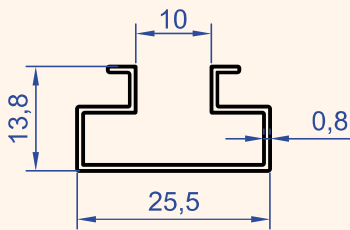
Profil No : 1068 Gramaj : 0.155 kg/m
