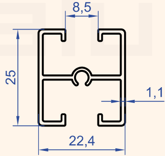
Profil No : 1910 Gramaj : 0.307 kg/m
