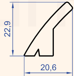
Profil No : 1285 Gramaj : 0.428 kg/m
