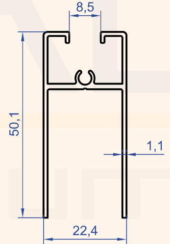
Profil No : 1914 Gramaj : 0.441 kg/m
