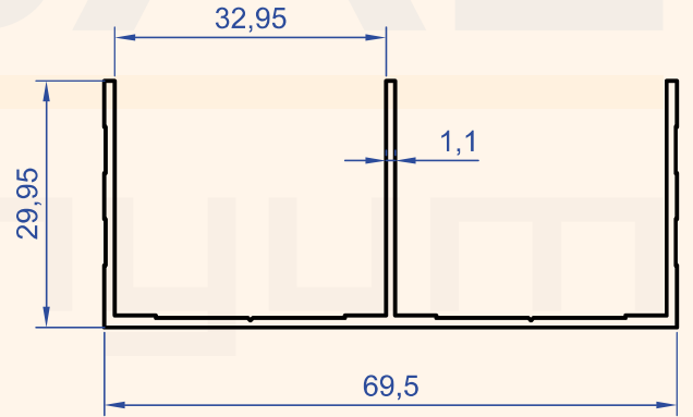
Profil No : 4834 Gramaj : 0.504 kg/m
