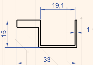
Profil No : 6922 Gramaj : 0.263 kg/m
