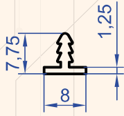
Profil No : 1211 Gramaj : 0.063 kg/m
