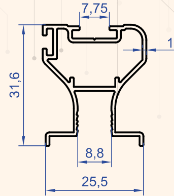
Profil No : 6758 Gramaj : 0.377 kg/m
