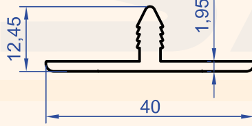
Profil No : 7275 Gramaj : 0.320 kg/m
