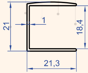
Profil No : 6316 Gramaj : 0.190 kg/m
