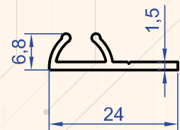
Profil No : 6883 Gramaj : 0.138 kg/m
