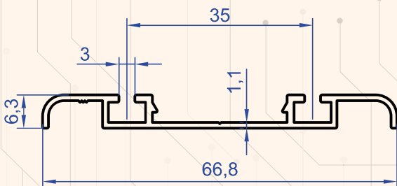
Profil No : 6903 Gramaj : 0.325 kg/m
