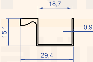
Profil No : 7507 Gramaj : 0.190 kg/m
