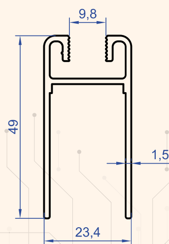
Profil No : 4932 Gramaj : 0.575 kg/m
