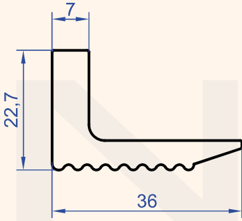
Profil No : 9569 Gramaj : 0.776 kg/m
