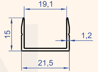
Profil No : 6923 Gramaj : 0.149 kg/m
