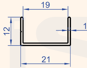
Profil No : 8944 Gramaj : 0.115 kg/m
