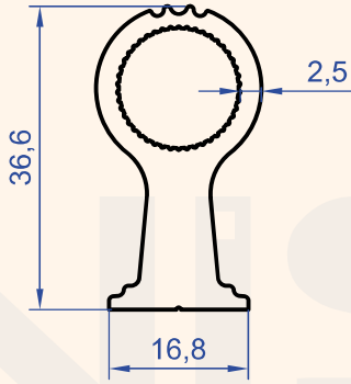
Profil No : 1166 Gramaj : 0.807 kg/m
