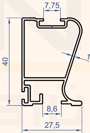
Profil No : 6420 Gramaj : 0.472 kg/m
