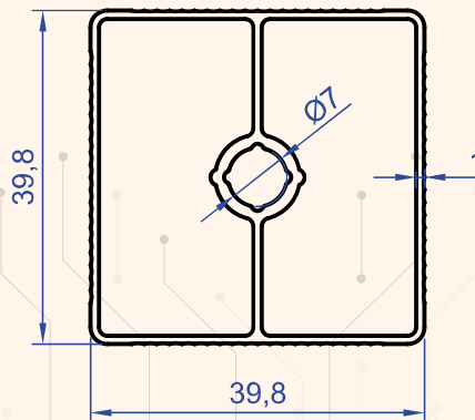
Profil No : 8766 Gramaj : 0.600 kg/m
