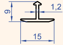
Profil No : 4642 Gramaj : 0.073 kg/m
