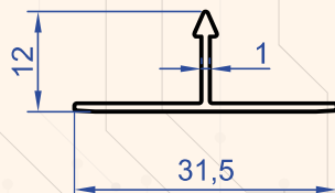
Profil No : 7332 Gramaj : 0.119 kg/m
