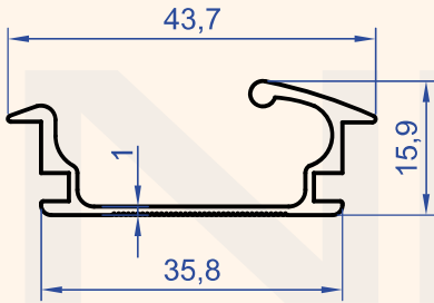
Profil No : 8975 Gramaj : 0.297 kg/m
