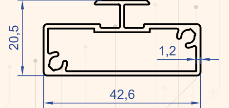
Profil No : 1931 Gramaj : 0.481 kg/m
