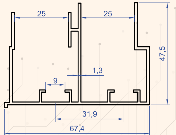
Profil No : 6939 Gramaj : 0.889 kg/m
