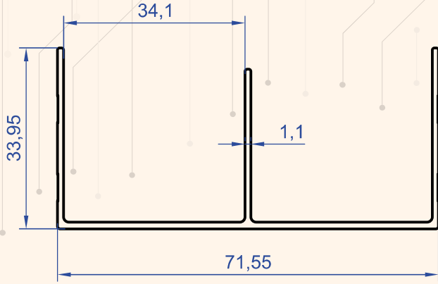
Profil No : 1303 Gramaj : 0.520 kg/m
