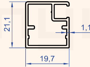
Profil No : 4501 Gramaj : 0.278 kg/m
