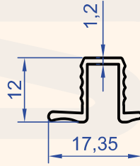
Profil No : 6878 Gramaj : 0.119 kg/m
