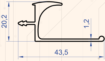
Profil No : 9086 Gramaj : 0.345 kg/m
