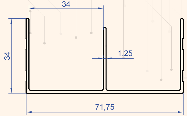
Profil No : 6919 Gramaj : 0.553 kg/m
