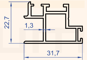
Profil No : 1188 Gramaj : 0.410 kg/m
