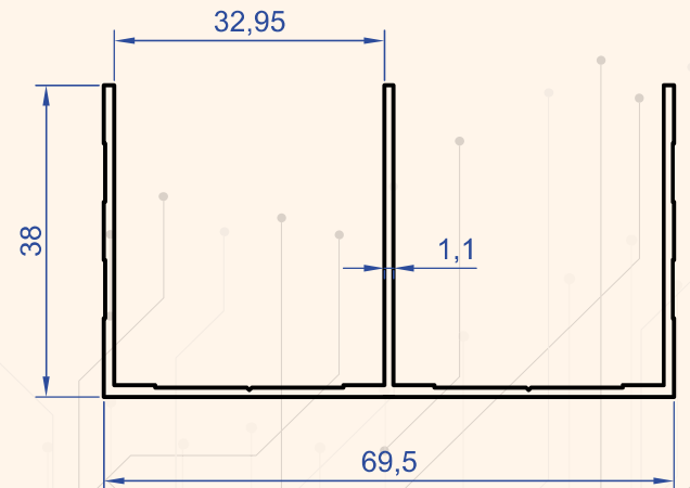
Profil No : 4841 Gramaj : 0.580 kg/m
