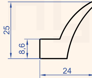
Profil No : 9290 Gramaj : 0.509 kg/m
