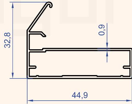
Profil No : 1132 Gramaj : 0.379 kg/m
