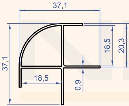
Profil No : 1333 Gramaj : 0.295 kg/m
