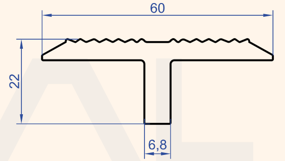
Profil No : 1134 Gramaj : 1.050 kg/m
