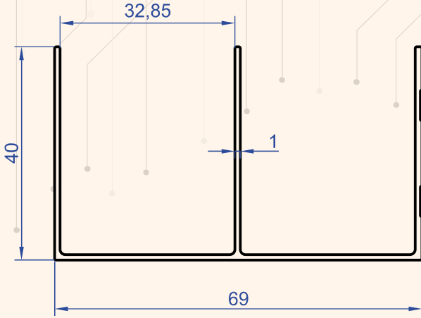
Profil No : 4629 Gramaj : 0.525 kg/m
