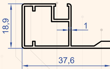
Profil No : 6857 Gramaj : 0.309 kg/m
