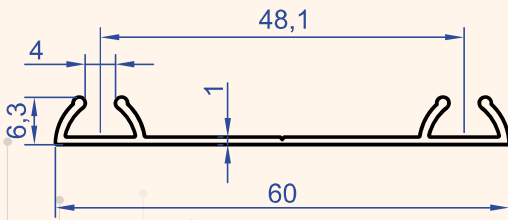
Profil No : 6884 Gramaj : 0.244 kg/m
