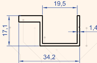
Profil No : 6188 Gramaj : 0.325 kg/m
