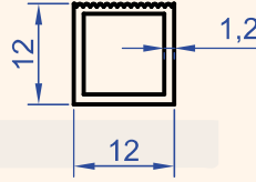
Profil No : 6299 Gramaj : 0.136 kg/m
