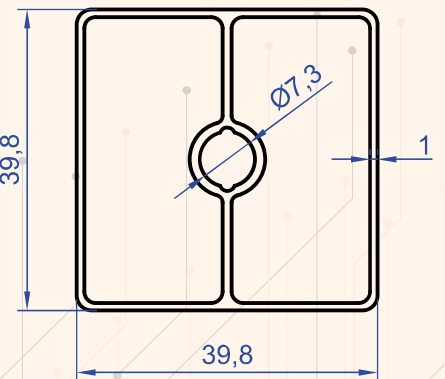
Profil No : 6332 Gramaj : 0.610 kg/m
