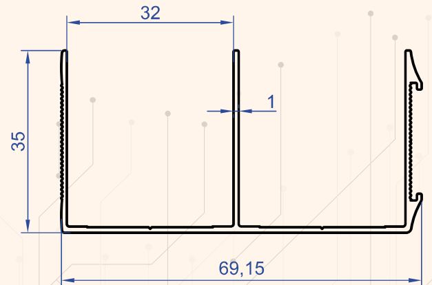
Profil No : 7499 Gramaj : 0.499 kg/m
