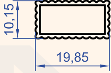
Profil No : 9174 Gramaj : 0.156 kg/m
