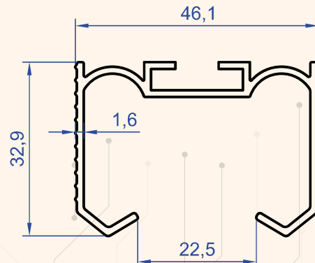
Profil No : 1383 Gramaj : 0.543 kg/m
