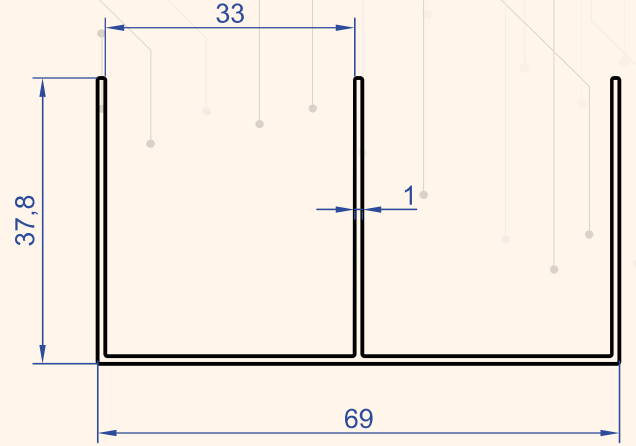
Profil No : 6307 Gramaj : 0.545 kg/m
