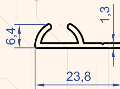
Profil No : 4830 Gramaj : 0.133 kg/m
