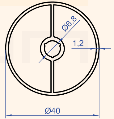
Profil No : 6333 Gramaj : 0.604 kg/m
