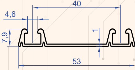
Profil No : 1041 Gramaj : 0.285 kg/m
