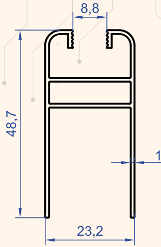
Profil No : 1171 Gramaj : 0.425 kg/m
