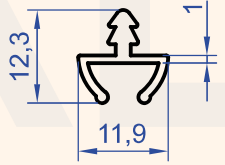
Profil No : 6877 Gramaj : 0.117 kg/m
