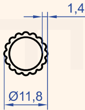
Profil No : 1031 Gramaj : 0.102 kg/m
