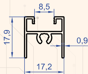
Profil No : 7523 Gramaj : 0.187 kg/m
