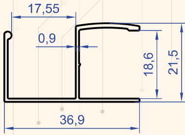
Profil No : 8927 Gramaj : 0.243 kg/m
