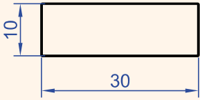
Profil No : 1214 Gramaj : 0.813 kg/m
