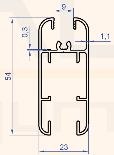
Profil No : 6484 Gramaj : 0.572 kg/m
