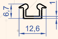
Profil No : 1032 Gramaj : 0.076 kg/m
