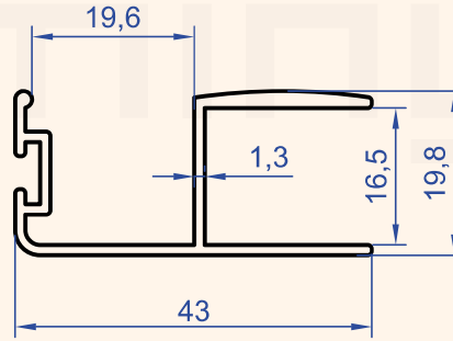
Profil No : 6864 Gramaj : 0.398 kg/m
