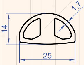
Profil No : 1129 Gramaj : 0.490 kg/m
