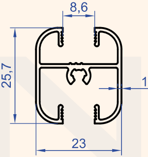
Profil No : 1172 Gramaj : 0.315 kg/m
