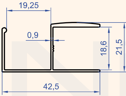
Profil No : 6308 Gramaj : 0.304 kg/m
