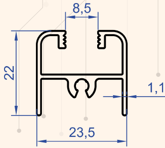
Profil No : 4621 Gramaj : 0.305 kg/m
