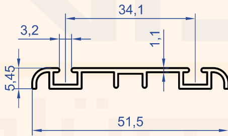
Profil No : 6723 Gramaj : 0.271 kg/m
