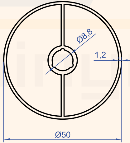
Profil No : 6737 Gramaj : 0.770 kg/m
