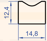
Profil No : 9581 Gramaj : 0.453 kg/m
