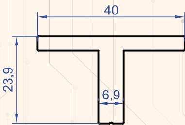
Profil No : 1071 Gramaj : 0.795 kg/m
