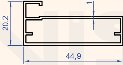
Profil No : 6854 Gramaj : 0.388 kg/m
