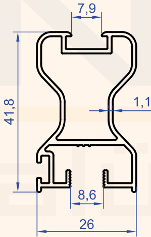
Profil No : 6302 Gramaj : 0.520 kg/m
