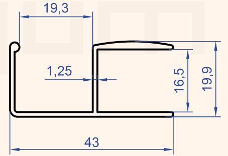
Profil No : 6866 Gramaj : 0.366 kg/m
