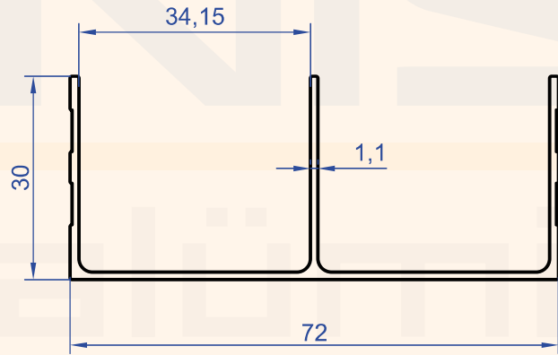
Profil No : 4491 Gramaj : 0.493 kg/m
