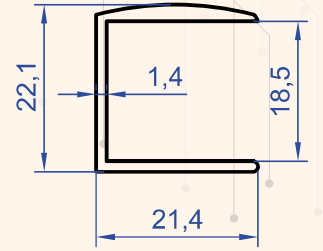
Profil No : 4309 Gramaj : 0.252 kg/m
