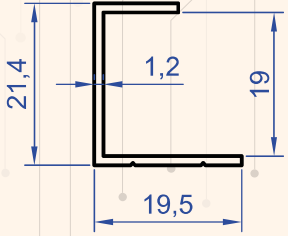
Profil No : 6187 Gramaj : 0.160 kg/m
