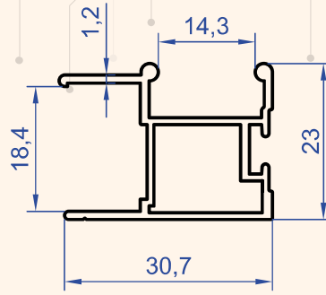
Profil No : 8631 Gramaj : 0.345 kg/m
