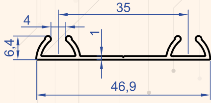
Profil No : 6873 Gramaj : 0.209 kg/m
