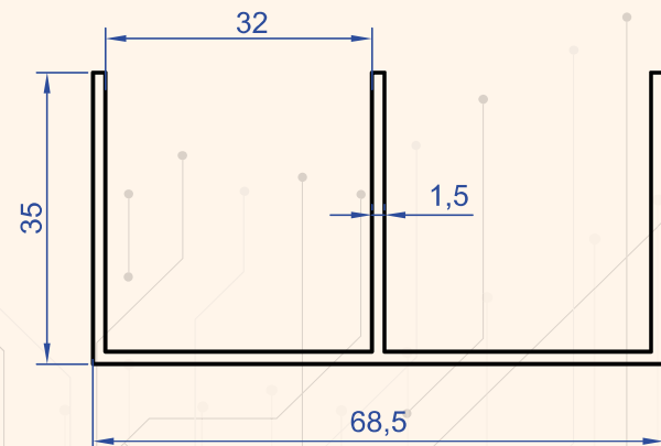
Profil No : 2842 Gramaj : 0.686 kg/m
