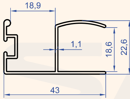
Profil No : 6717 Gramaj : 0.360 kg/m
