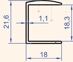
Profil No : 1164 Gramaj : 0.195 kg/m
