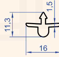
Profil No : T201 Gramaj : 0.145 kg/m
