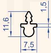
Profil No : 1210 Gramaj : 0.110 kg/m
