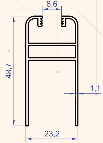
Profil No : 1986 Gramaj : 0.473 kg/m
