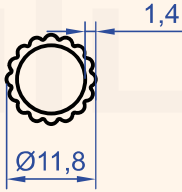
Profil No : 1031 Gramaj : 0.102 kg/m
