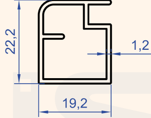
Profil No : 1934 Gramaj : 0.285 kg/m
