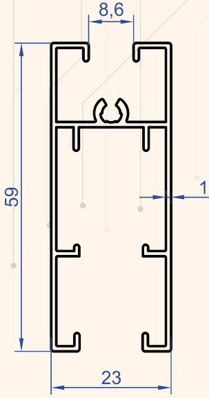
Profil No : 7501 Gramaj : 0.545 kg/m
