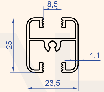
Profil No : 4630 Gramaj : 0.384 kg/m
