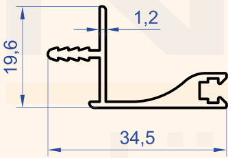
Profil No : 1127 Gramaj : 0.290 kg/m
