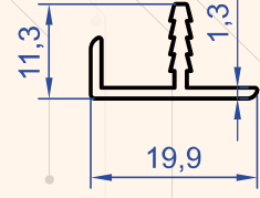
Profil No : 2655 Gramaj : 0.141 kg/m
