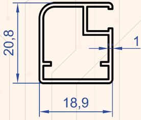
Profil No : 6858 Gramaj : 0.230 kg/m
