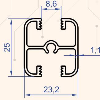
Profil No : 1984 Gramaj : 0.351 kg/m
