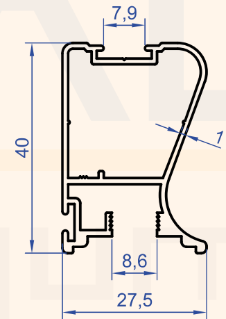
Profil No : 6443 Gramaj : 0.504 kg/m
