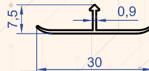
Profil No : 1341 Gramaj : 0.088 kg/m
