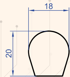
Profil No : 9507 Gramaj : 0.805 kg/m
