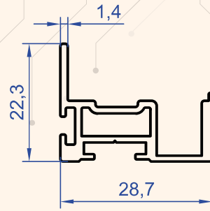
Profil No : 6764 Gramaj : 0.360 kg/m
