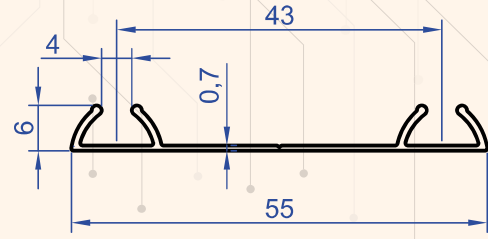
Profil No : 1039 Gramaj : 0.172 kg/m
