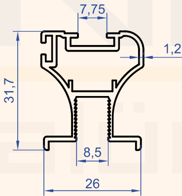
Profil No : 6838 Gramaj : 0.469 kg/m
