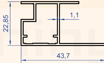
Profil No : 4312 Gramaj : 0.369 kg/m
