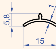
Profil No : 1343 Gramaj : 0.050 kg/m
