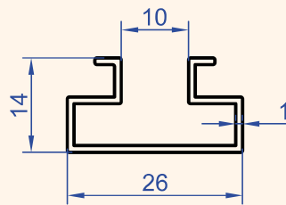
Profil No : 6791 Gramaj : 0.195 kg/m
