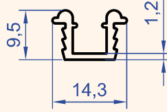
Profil No : 3090 Gramaj : 0.128 kg/m
