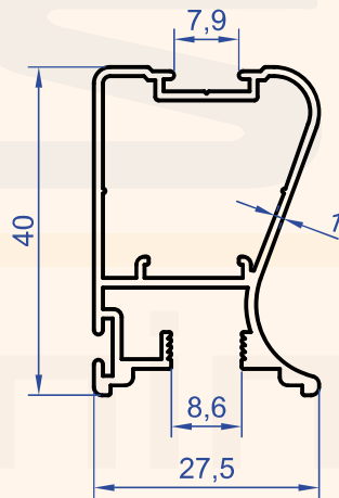
Profil No : 7240 Gramaj : 0.518 kg/m
