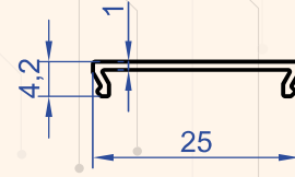
Profil No : 7497 Gramaj : 0.087 kg/m
