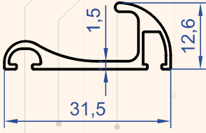
Profil No : 1072 Gramaj : 0.236 kg/m
