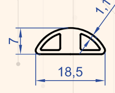
Profil No : 9631 Gramaj : 0.187 kg/m
