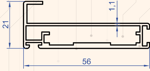
Profil No : 6890 Gramaj : 0.602 kg/m
