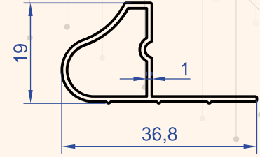
Profil No : 1277 Gramaj : 0.216 kg/m
