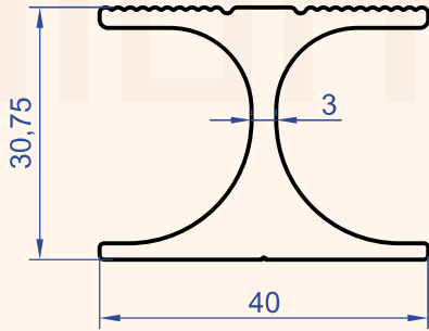
Profil No : 1169 Gramaj : 1.062 kg/m
