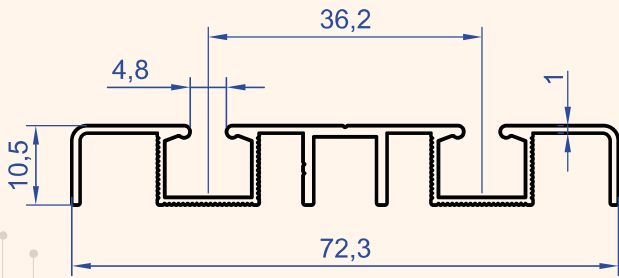
Profil No : 1258 Gramaj : 0.479 kg/m
