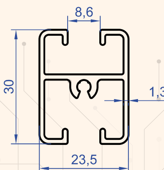
Profil No : 4623 Gramaj : 0.455 kg/m
