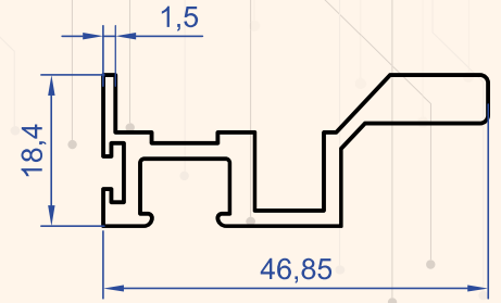
Profil No : 6898 Gramaj : 0.653 kg/m
