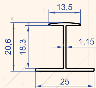
Profil No : 6106 Gramaj : 0.168 kg/m
