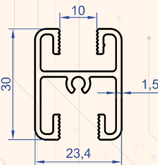
Profil No : 6195 Gramaj : 0.531 kg/m
