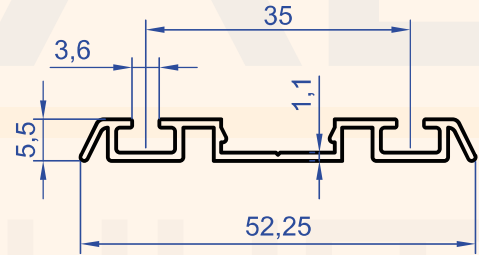
Profil No : 6869 Gramaj : 0.274 kg/m
