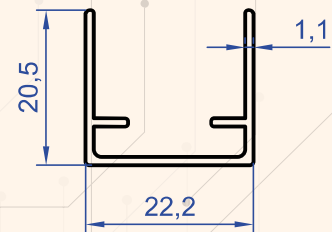
Profil No : 6820 Gramaj : 0.209 kg/m
