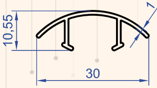
Profil No : 1305 Gramaj : 0.141 kg/m
