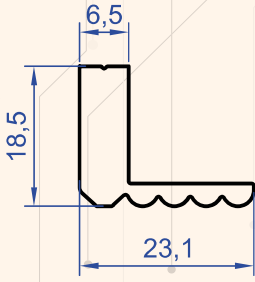
Profil No : 1334 Gramaj : 0.429 kg/m
