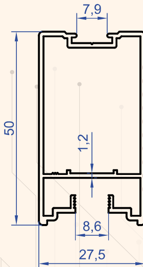
Profil No : 6902 Gramaj : 0.575 kg/m
