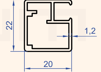
Profil No : 6462 Gramaj : 0.317 kg/m
