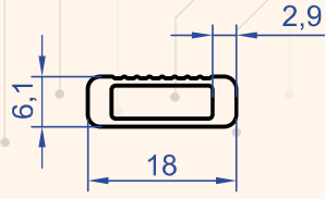
Profil No : 6769 Gramaj : 0.154 kg/m
