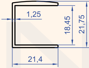
Profil No : 6867 Gramaj : 0.238 kg/m
