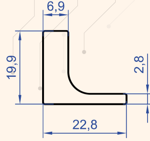
Profil No : 7339 Gramaj : 0.513 kg/m
