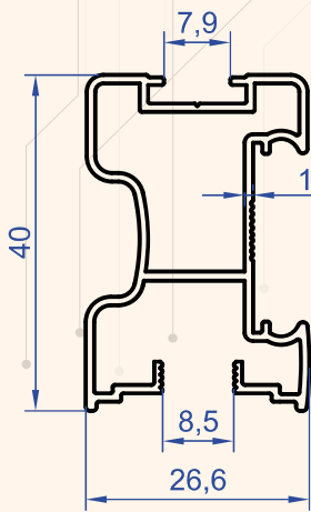
Profil No : 7500 Gramaj : 0.467 kg/m
