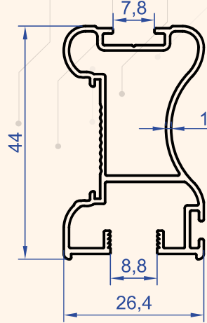
Profil No : 7225 Gramaj : 0.491 kg/m
