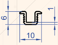
Profil No : 6879 Gramaj : 0.051 kg/m
