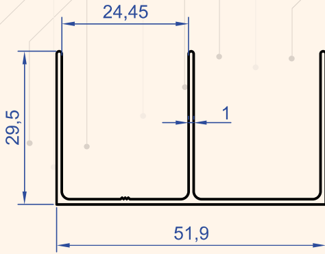
Profil No : 6442 Gramaj : 0.377 kg/m
