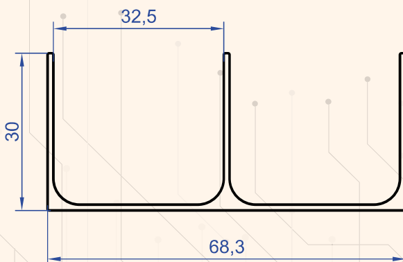
Profil No : 4114 Gramaj : 0.520 kg/m
