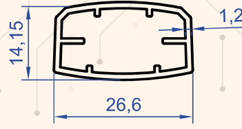
Profil No : 1130 Gramaj : 0.273 kg/m
