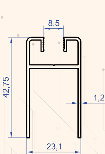
Profil No : 4835 Gramaj : 0.425 kg/m
