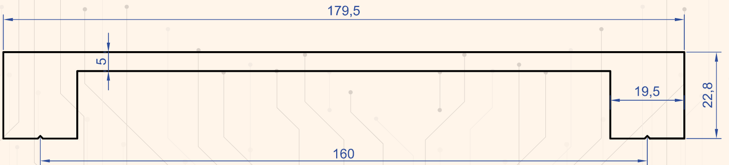
Profil No : 8751 Gramaj : 4.310 kg/m
