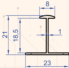
Profil No : 1165 Gramaj : 0.136 kg/m
