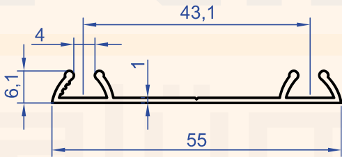
Profil No : 6306 Gramaj : 0.228 kg/m
