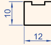
Profil No : 6422 Gramaj : 0.303 kg/m
