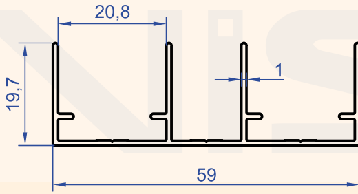
Profil No : 6108 Gramaj : 0.382 kg/m
