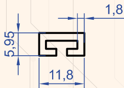
Profil No : 1256 Gramaj : 0.129 kg/m
