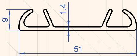
Profil No : 4631 Gramaj : 0.349 kg/m
