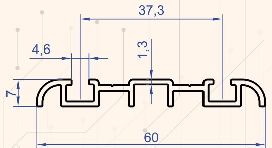
Profil No : 4634 Gramaj : 0.391 kg/m
