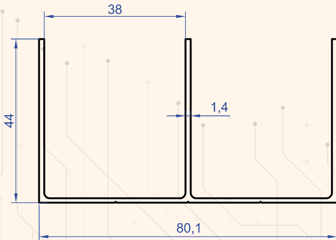
Profil No : 6870 Gramaj : 0.745 kg/m
