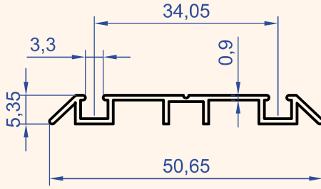
Profil No : 1200 Gramaj : 0.211 kg/m
