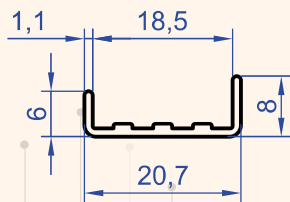
Profil No : 2631 Gramaj : 0.106 kg/m
