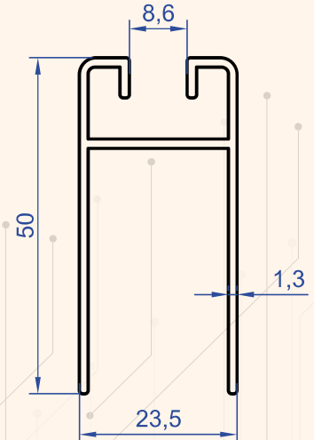
Profil No : 4628 Gramaj : 0.506 kg/m
