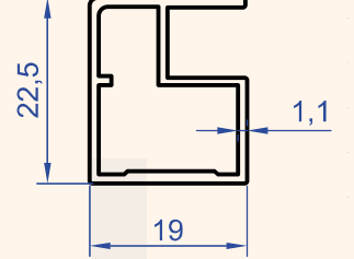
Profil No : 3983 Gramaj : 0.276 kg/m
