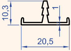
Profil No : 3177 Gramaj : 0.119 kg/m
