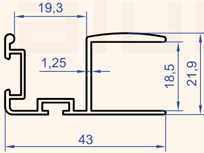
Profil No : 6861 Gramaj : 0.420 kg/m
