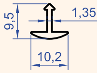
Profil No : 4649 Gramaj : 0.068 kg/m
