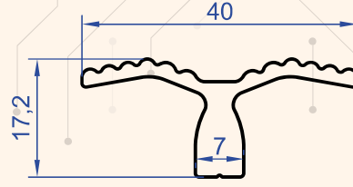
Profil No : 1346 Gramaj : 0.440 kg/m
