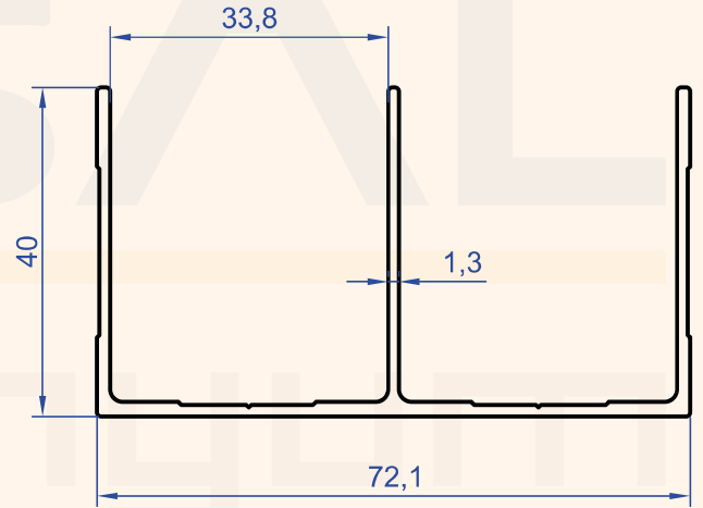
Profil No : 4629 Gramaj : 0.752 kg/m
