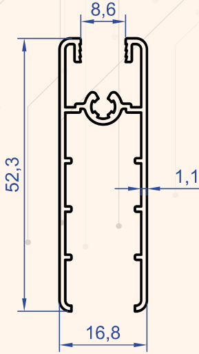
Profil No : 4948 Gramaj : 0.447 kg/m
