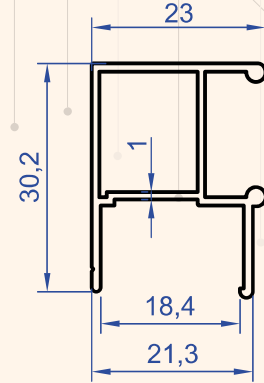
Profil No : 8994 Gramaj : 0.316 kg/m
