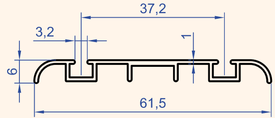
Profil No : 6115 Gramaj : 0.282 kg/m
