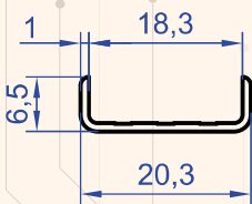
Profil No : 6314 Gramaj : 0.078 kg/m
