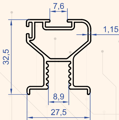
Profil No : 6432 Gramaj : 0.458 kg/m
