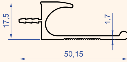
Profil No : 4564 Gramaj : 0.456 kg/m
