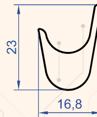
Profil No : 9632 Gramaj : 0.410 kg/m
