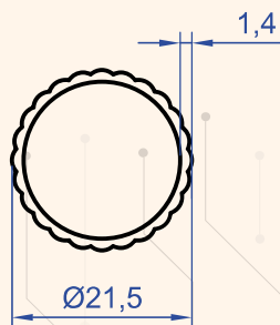
Profil No : 6905 Gramaj : 0.214 kg/m
