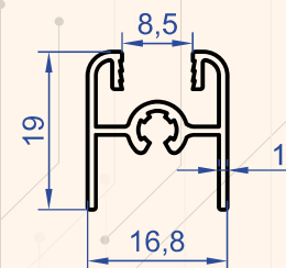
Profil No : 4947 Gramaj : 0.211 kg/m
