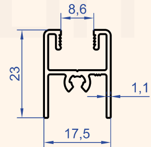
Profil No : 6900 Gramaj : 0.266 kg/m
