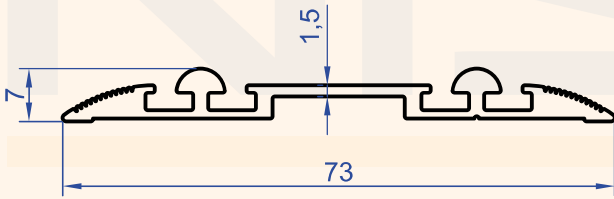
Profil No : 6196 Gramaj : 0.509 kg/m
