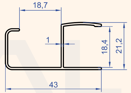
Profil No : 1152 Gramaj : 0.272 kg/m
