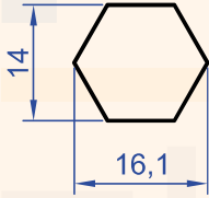
Profil No : 161 Gramaj : 0.458 kg/m
