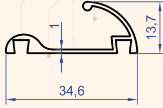
Profil No : 8691 Gramaj : 0.217 kg/m
