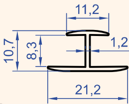
Profil No : T1528 Gramaj : 0.115 kg/m
