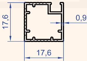
Profil No : 1291 Gramaj : 0.188 kg/m
