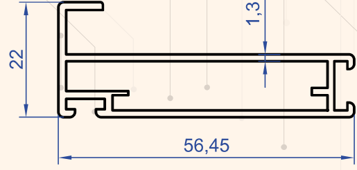
Profil No : 2668 Gramaj : 0.594 kg/m
