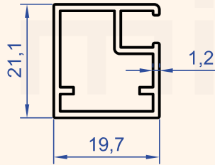
Profil No : 6860 Gramaj : 0.295 kg/m
