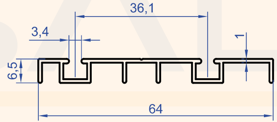
Profil No : 1259 Gramaj : 0.309 kg/m
