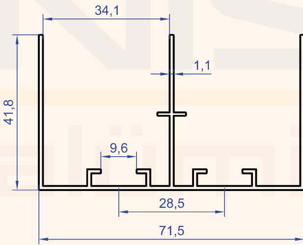
Profil No : 7430 Gramaj : 0.678 kg/m
