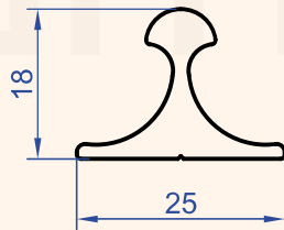
Profil No : 1253 Gramaj : 0.363 kg/m
