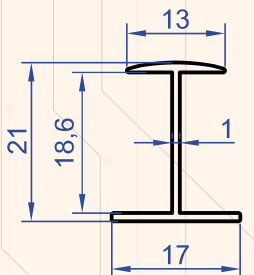
Profil No : 1059 Gramaj : 0.137 kg/m
