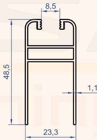
Profil No : 4493 Gramaj : 0.476 kg/m
