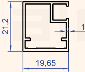
Profil No : 6749 Gramaj : 0.263 kg/m
