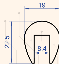
Profil No : 6166 Gramaj : 0.605 kg/m
