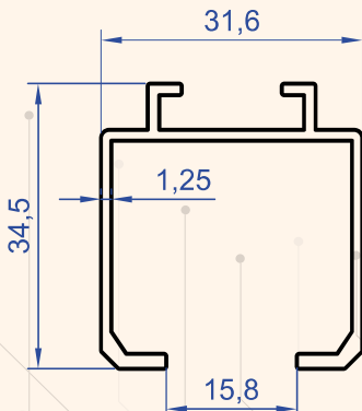
Profil No : 8554 Gramaj : 0.425 kg/m
