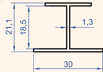
Profil No : 1999 Gramaj : 0.241 kg/m
