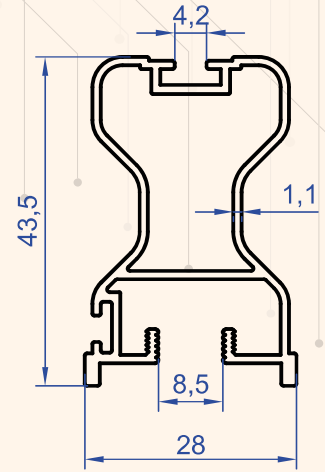
Profil No : 4496 Gramaj : 0.554 kg/m
