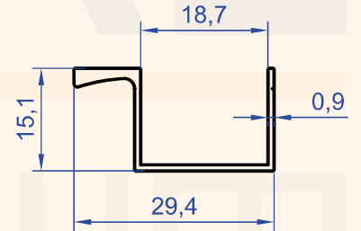
Profil No : 8926 Gramaj : 0.166 kg/m
