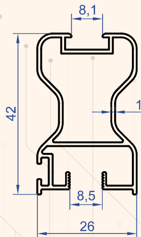
Profil No : 6713 Gramaj : 0.472 kg/m
