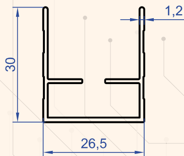
Profil No : 6924 Gramaj : 0.309 kg/m
