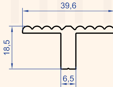
Profil No : 1179 Gramaj : 0.546 kg/m
