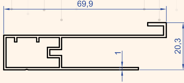
Profil No : 1192 Gramaj : 0.497 kg/m
