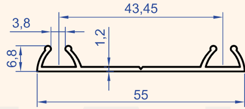
Profil No : 4829 Gramaj : 0.257 kg/m
