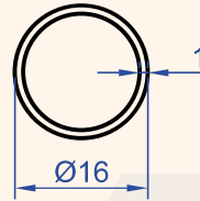
Profil No : 1062 Gramaj : 0.138 kg/m
