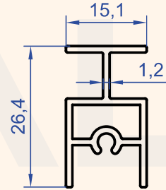
Profil No : 1176 Gramaj : 0.290 kg/m
