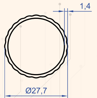
Profil No : 6904 Gramaj : 0.282 kg/m
