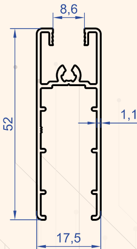
Profil No : 6496 Gramaj : 0.439 kg/m
