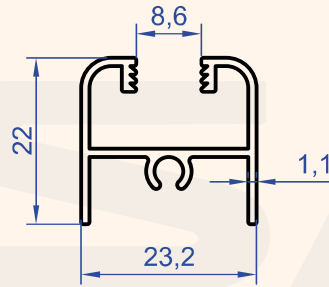
Profil No : 1985 Gramaj : 0.280 kg/m
