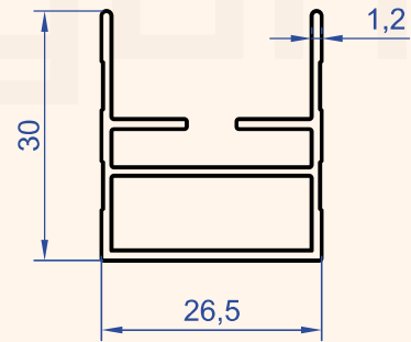
Profil No : 6925 Gramaj : 0.385 kg/m
