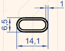
Profil No : 7380 Gramaj : 0.081 kg/m
