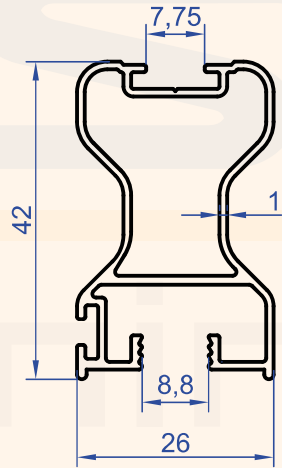
Profil No : 6752 Gramaj : 0.485 kg/m
