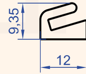
Profil No : 1366 Gramaj : 0.184 kg/m
