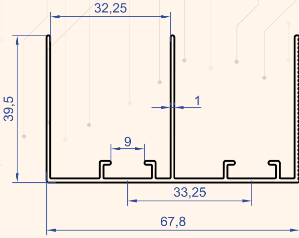
Profil No : 1113 Gramaj : 0.550 kg/m
