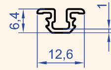
Profil No : 4912 Gramaj : 0.073 kg/m
