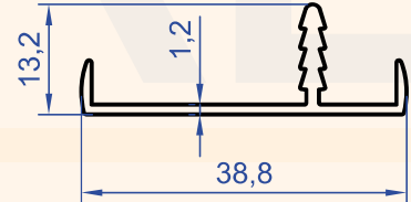
Profil No : 6715 Gramaj : 0.225 kg/m
