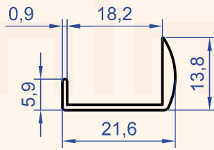
Profil No : 4944 Gramaj : 0.133 kg/m
