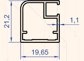
Profil No : 4474 Gramaj : 0.265 kg/m
