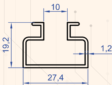
Profil No : 3800 Gramaj : 0.274 kg/m
