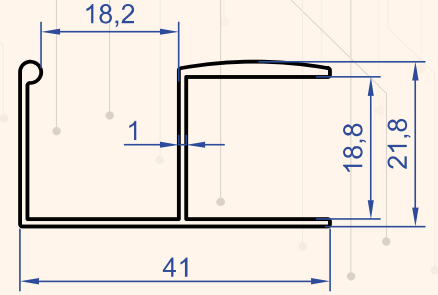
Profil No : 6317 Gramaj : 0.320 kg/m
