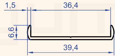
Profil No : 6753 Gramaj : 0.171 kg/m
