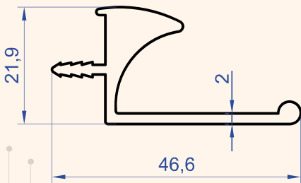
Profil No : 6390 Gramaj : 0.609 kg/m
