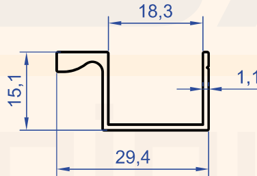
Profil No : 6706 Gramaj : 0.217 kg/m
