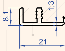
Profil No : 4498 Gramaj : 0.150 kg/m
