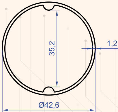
Profil No : 1006 Gramaj : 0.475 kg/m
