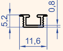
Profil No : 7521 Gramaj : 0.054 kg/m
