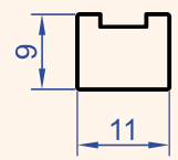
Profil No : 8743 Gramaj : 0.245 kg/m
