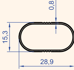
Profil No : 1004 Gramaj : 0.145 kg/m
