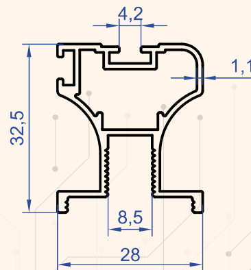
Profil No : 4495 Gramaj : 0.469 kg/m
