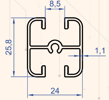
Profil No : 4492 Gramaj : 0.370 kg/m
