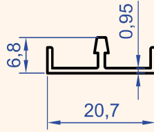
Profil No : 6055 Gramaj : 0.101 kg/m
