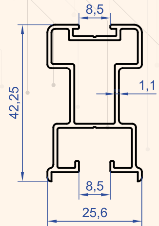
Profil No : 1911 Gramaj : 0.496 kg/m
