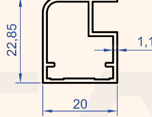
Profil No : 4311 Gramaj : 0.268 kg/m
