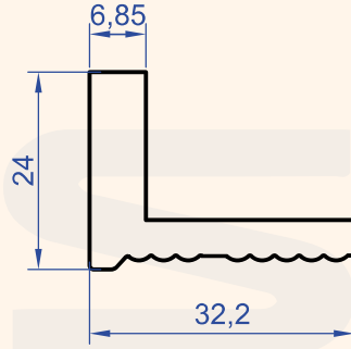
Profil No : 1218 Gramaj : 0.755 kg/m
