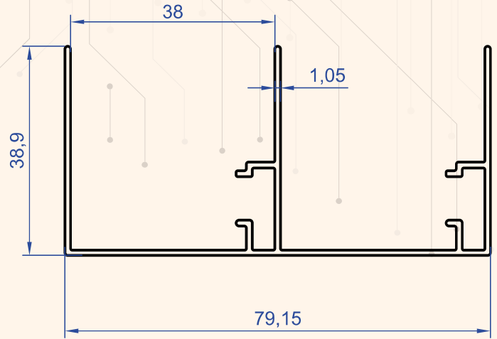
Profil No : 1040 Gramaj : 0.623 kg/m
