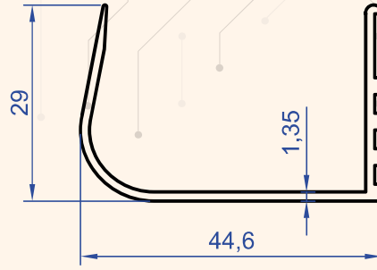
Profil No : 1350 Gramaj : 0.369 kg/m
