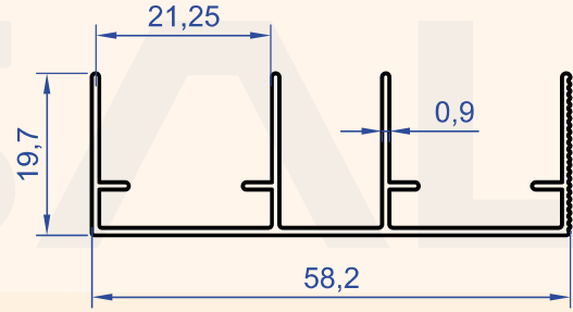
Profil No : 1025 Gramaj : 0.357 kg/m
