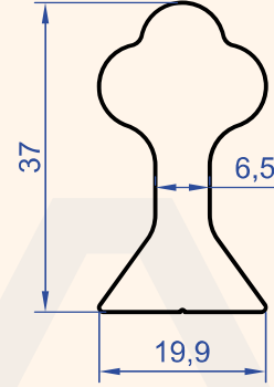
Profil No : 1167 Gramaj : 1.194 kg/m
