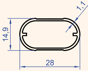
Profil No : 9104 Gramaj : 0.203 kg/m
