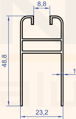
Profil No : 6325 Gramaj : 0.436 kg/m
