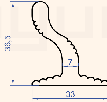
Profil No : 1384 Gramaj : 0.900 kg/m
