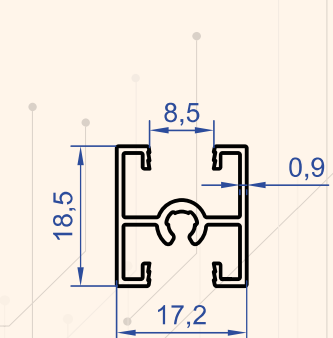
Profil No : 7524 Gramaj : 0.217 kg/m
