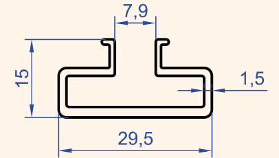
Profil No : 1925 Gramaj : 0.332 kg/m
