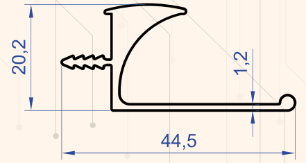
Profil No : 6421 Gramaj : 0.417 kg/m
