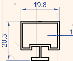
Profil No : 1190 Gramaj : 0.237 kg/m
