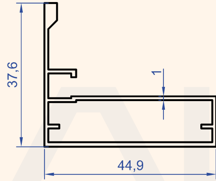
Profil No : 6889 Gramaj : 0.469 kg/m
