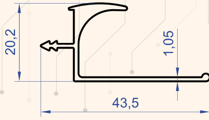
Profil No : 1097 Gramaj : 0.295 kg/m
