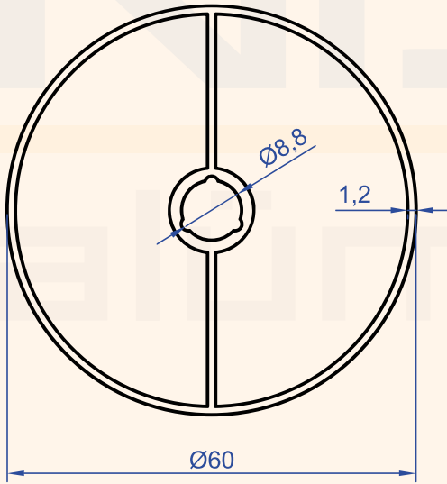
Profil No : 6738 Gramaj : 0.902 kg/m
