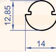
Profil No : 6400 Gramaj : 0.344 kg/m
