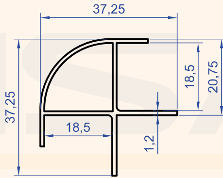
Profil No : 6107 Gramaj : 0.360 kg/m
