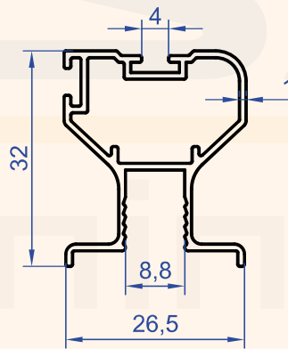
Profil No : 6414 Gramaj : 0.371 kg/m
