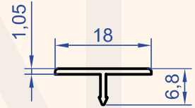
Profil No : 1323 Gramaj : 0.066 kg/m
