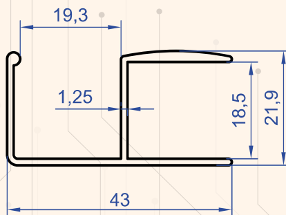
Profil No : 6868 Gramaj : 0.379 kg/m
