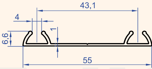
Profil No : 6824 Gramaj : 0.230 kg/m
