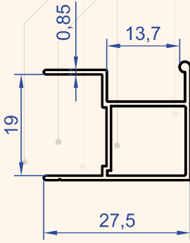
Profil No : 1046 Gramaj : 0.226 kg/m
