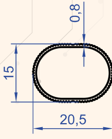
Profil No : 1003 Gramaj : 0.106 kg/m
