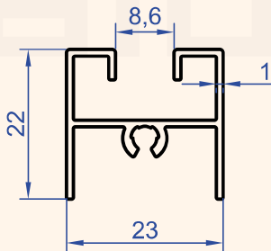
Profil No : 7503 Gramaj : 0.263 kg/m
