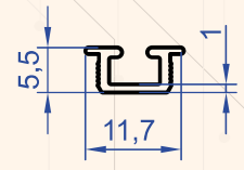
Profil No : 6931 Gramaj : 0.070 kg/m
