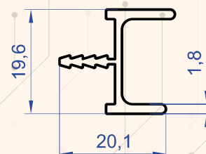
Profil No : 4565 Gramaj : 0.225 kg/m
