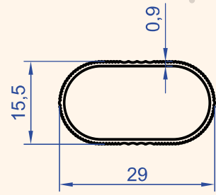
Profil No : 7330 Gramaj : 0.160 kg/m
