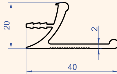
Profil No : 1907 Gramaj : 0.446 kg/m
