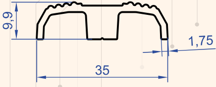
Profil No : 1348 Gramaj : 0.400 kg/m
