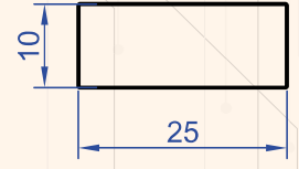
Profil No : 5 Gramaj : 0.677 kg/m
