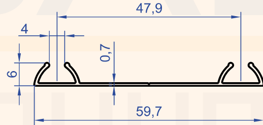
Profil No : 1036 Gramaj : 0.175 kg/m
