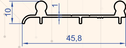
Profil No : 6304 Gramaj : 0.293 kg/m
