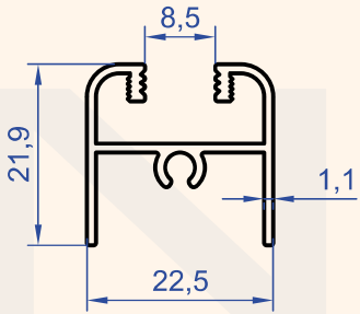
Profil No : 6719 Gramaj : 0.279 kg/m
