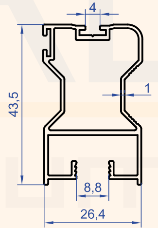
Profil No : 6985 Gramaj : 0.523 kg/m
