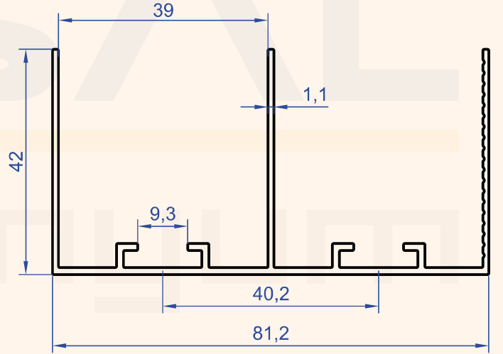
Profil No : 7428 Gramaj : 0.743 kg/m
