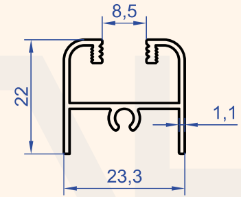
Profil No : 4494 Gramaj : 0.285 kg/m
