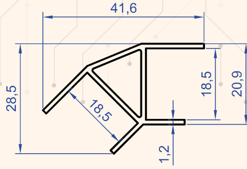
Profil No : 1909 Gramaj : 0.377 kg/m
