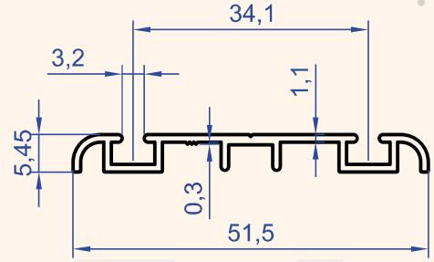
Profil No : 6497 Gramaj : 0.271 kg/m
