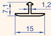
Profil No : 1342 Gramaj : 0.067 kg/m
