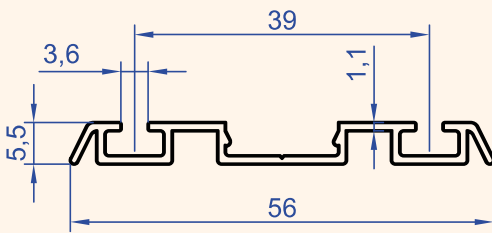
Profil No : 6872 Gramaj : 0.284 kg/m
