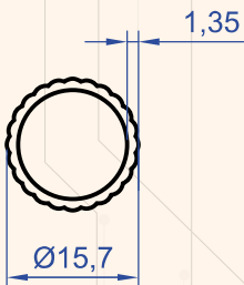
Profil No : 6906 Gramaj : 0.152 kg/m
