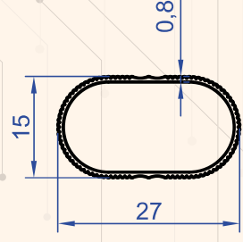
Profil No : 1028 Gramaj : 0.133 kg/m
