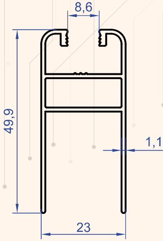
Profil No : 6300 Gramaj : 0.480 kg/m
