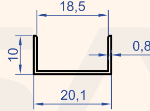
Profil No : 1066 Gramaj : 0.085 kg/m
