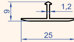
Profil No : 1302 Gramaj : 0.103 kg/m
