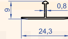
Profil No : 1008 Gramaj : 0.075 kg/m
