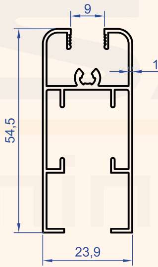
Profil No : 6822 Gramaj : 0.537 kg/m
