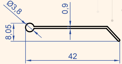
Profil No : 1075 Gramaj : 0.130 kg/m
