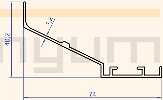
Profil No : 1124 Gramaj : 0.396 kg/m
