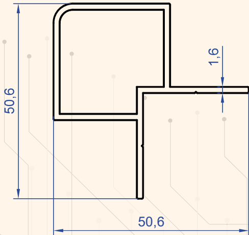
Profil No : 1355 Gramaj : 0.664 kg/m
