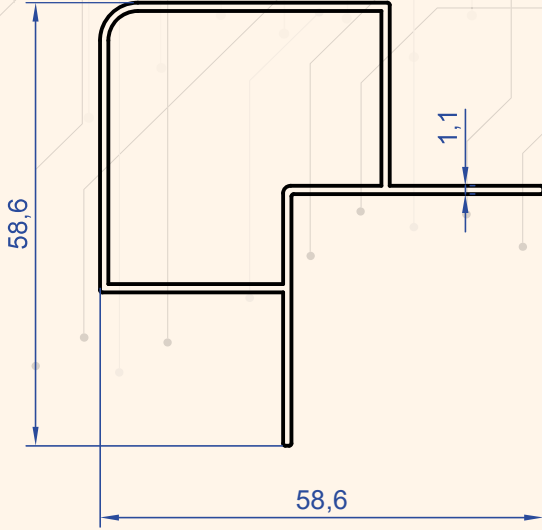
Profil No : 1295 Gramaj : 0.558 kg/m
