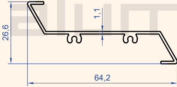
Profil No : 1391 Gramaj : 0.354 kg/m
