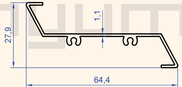
Profil No : 1298 Gramaj : 0.355 kg/m
