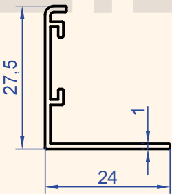
Profil No : 1328 Gramaj : 0.170 kg/m
