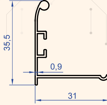
Profil No : 1143 Gramaj : 0.232 kg/m
