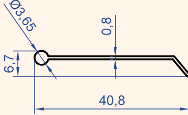
Profil No : 1145 Gramaj : 0.113 kg/m
