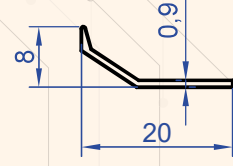
Profil No : 1262 Gramaj : 0.058 kg/m
