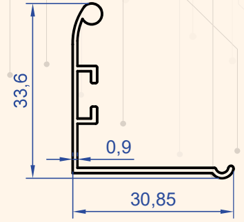
Profil No : 1147 Gramaj : 0.227 kg/m
