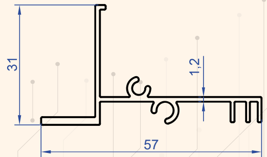
Profil No : 1227 Gramaj : 0.430 kg/m
