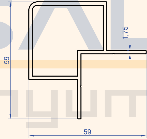
Profil No : 1356 Gramaj : 0.892 kg/m
