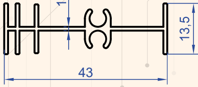
Profil No : 1330 Gramaj : 0.322 kg/m
