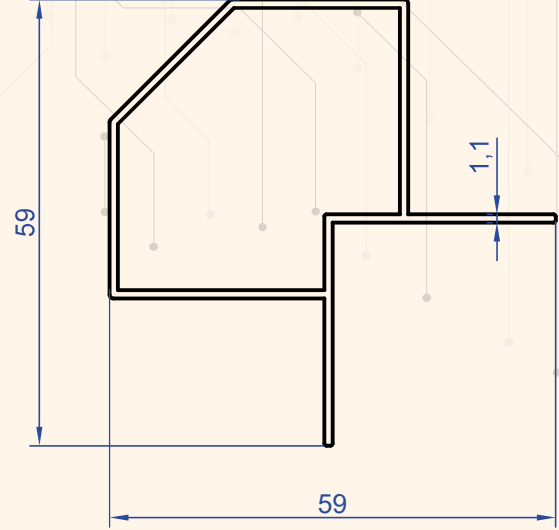
Profil No : 1297 Gramaj : 0.547 kg/m
