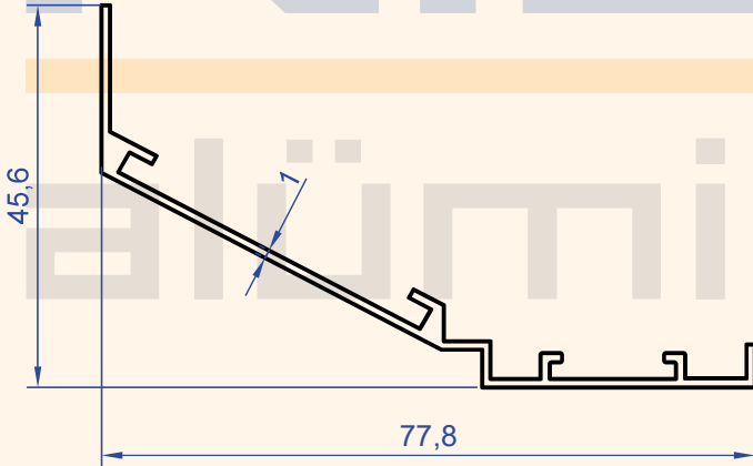
Profil No : 1236 Gramaj : 0.391 kg/m
