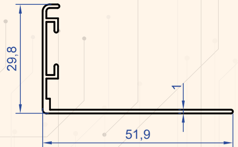
Profil No : 1074 Gramaj : 0.266 kg/m
