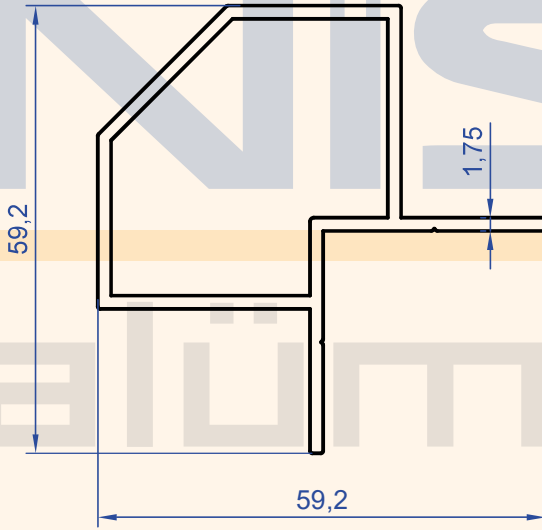
Profil No : 1357 Gramaj : 0.862 kg/m
