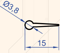
Profil No : 1149 Gramaj : 0.063 kg/m
