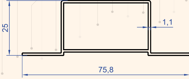
Profil No : 1304 Gramaj : 0.481 kg/m
