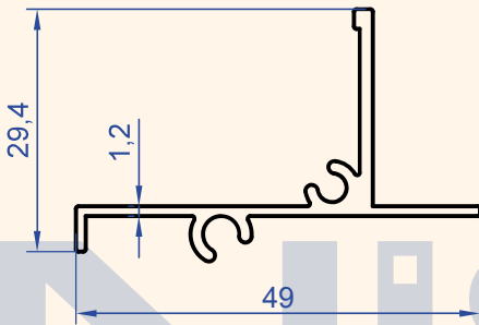
Profil No : 1144 Gramaj : 0.365 kg/m
