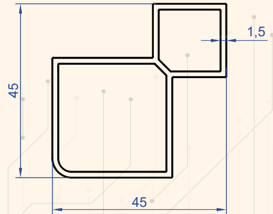
Profil No : 1261 Gramaj : 0.712 kg/m
