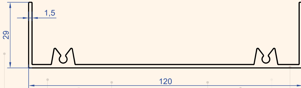
Profil No : 1225 Gramaj : 0.940 kg/m
