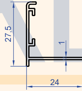
Profil No : 1327 Gramaj : 0.168 kg/m
