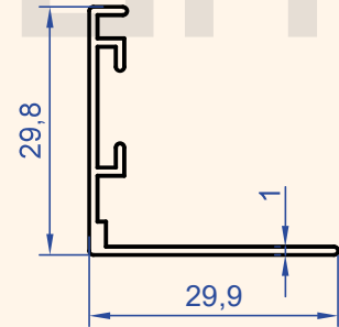
Profil No : 1087 Gramaj : 0.209 kg/m
