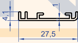
Profil No : 1320 Gramaj : 0.120 kg/m
