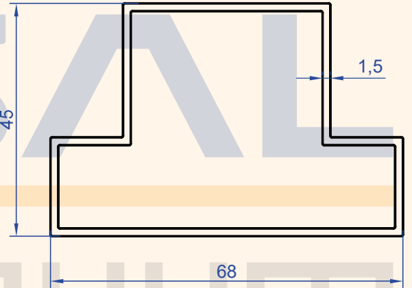
Profil No : 1260 Gramaj : 0.894 kg/m
