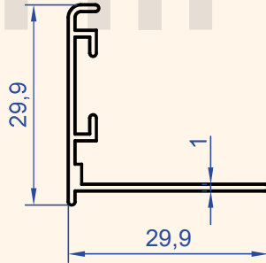
Profil No : 1086 Gramaj : 0.206 kg/m
