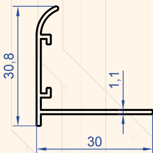
Profil No : 1148 Gramaj : 0.206 kg/m
