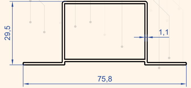
Profil No : 1294 Gramaj : 0.507 kg/m
