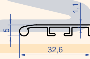
Profil No : 1319 Gramaj : 0.165 kg/m
