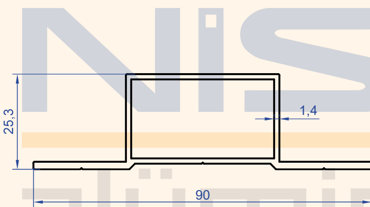
Profil No : 1354 Gramaj : 0.748 kg/m
