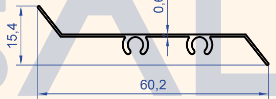
Profil No : 1146 Gramaj : 0.180 kg/m
