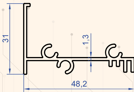
Profil No : 1088 Gramaj : 0.455 kg/m
