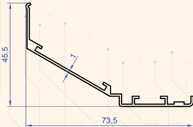
Profil No : 1085 Gramaj : 0.387 kg/m
