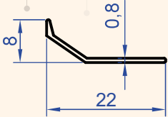
Profil No : 1318 Gramaj : 0.056 kg/m
