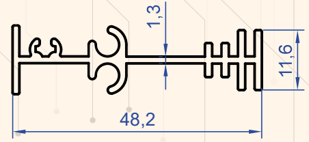
Profil No : 1089 Gramaj : 0.442 kg/m
