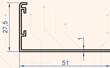
Profil No : 1329 Gramaj : 0.241 kg/m
