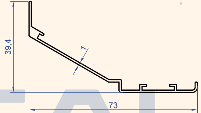
Profil No : 1332 Gramaj : 0.330 kg/m
