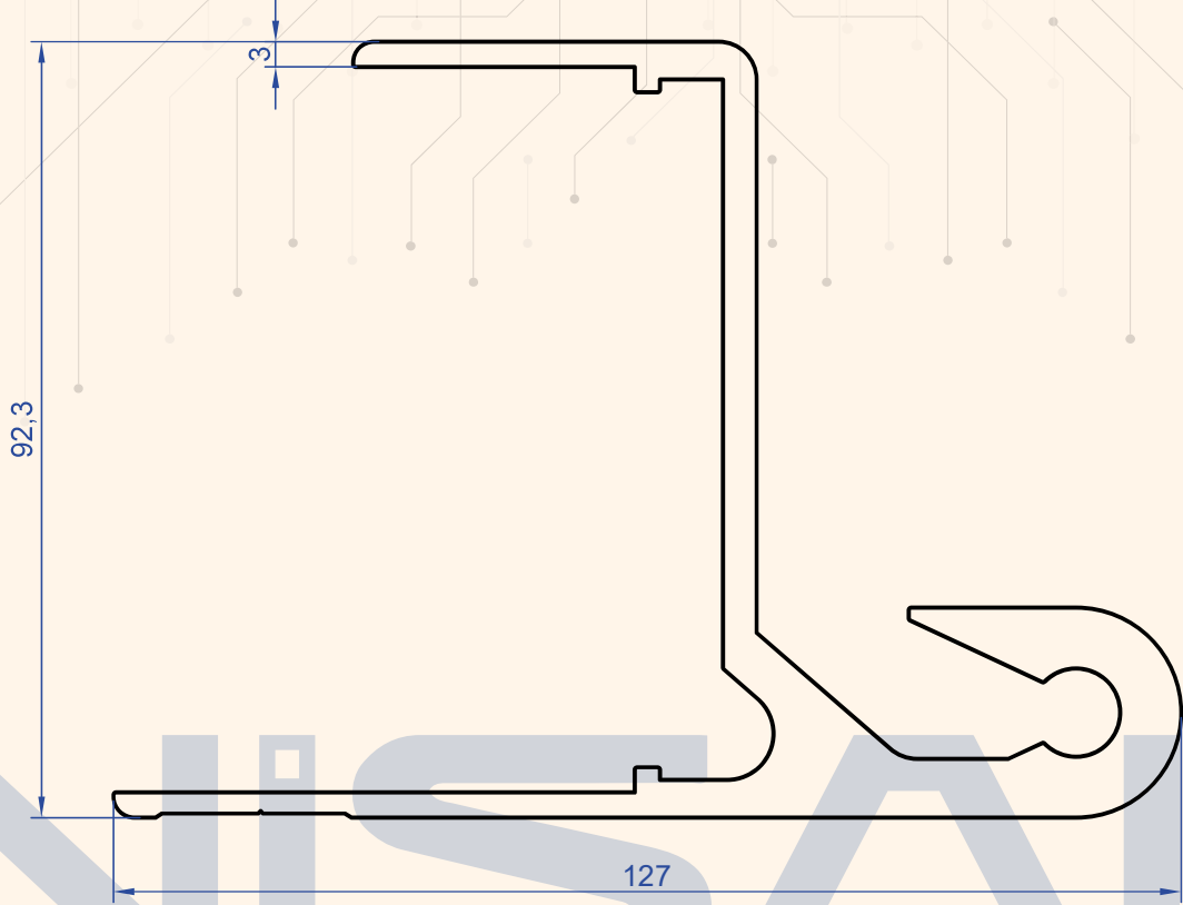
Profil No : 2710 Gramaj : 3.802 kg/m
