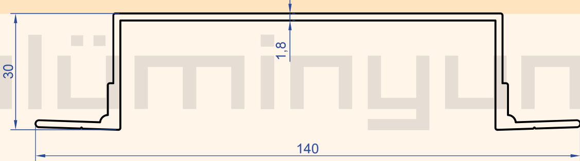
Profil No : 2663 Gramaj : 1.047 kg/m
