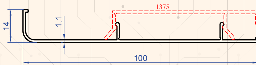
Profil No : 1376 Gramaj : 0.379 kg/m
