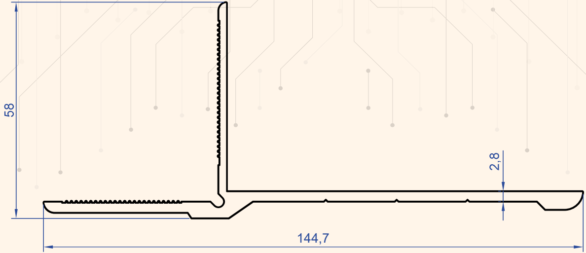
Profil No : 2711 Gramaj : 1.545 kg/m
