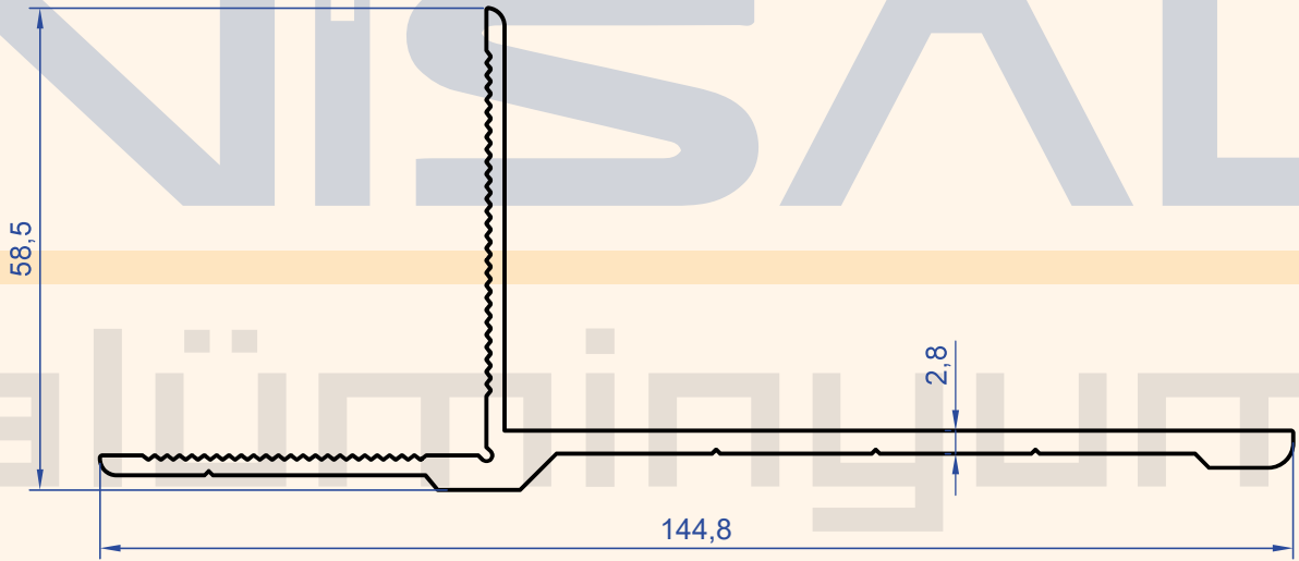
Profil No : 4168 Gramaj : 1.444 kg/m
