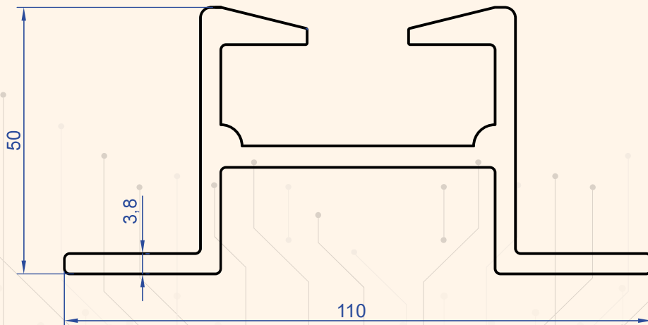
Profil No : 1955 Gramaj : 2.614 kg/m
