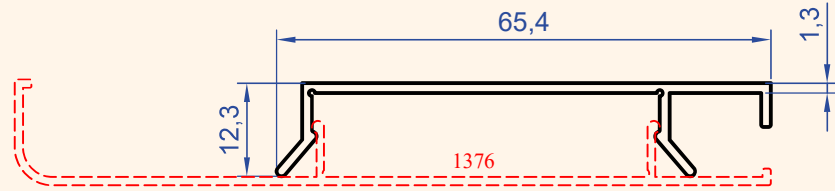
Profil No : 1375 Gramaj : 0.320 kg/m
