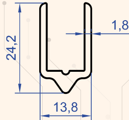
Profil No : 1338 Gramaj : 0.285 kg/m
