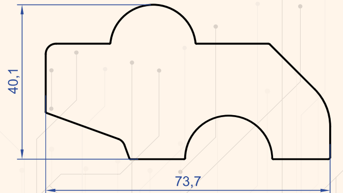
Profil No : 1121 Gramaj : 5.088 kg/m
