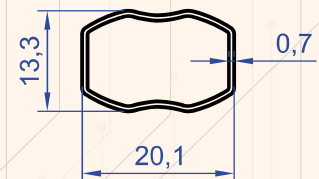
Profil No : 1223 Gramaj : 0.107 kg/m
