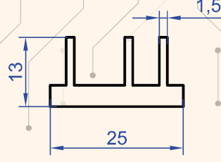
Profil No : 8991 Gramaj : 0.417 kg/m
