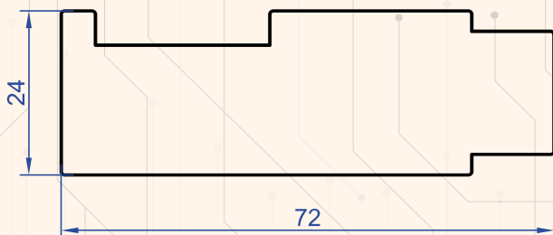
Profil No : 1237 Gramaj : 4.140 kg/m
