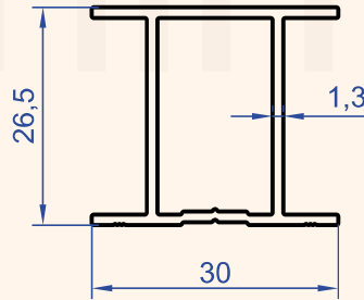
Profil No : 1215 Gramaj : 0.379 kg/m
