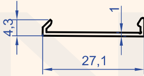
Profil No : 8578 Gramaj : 0.095 kg/m
