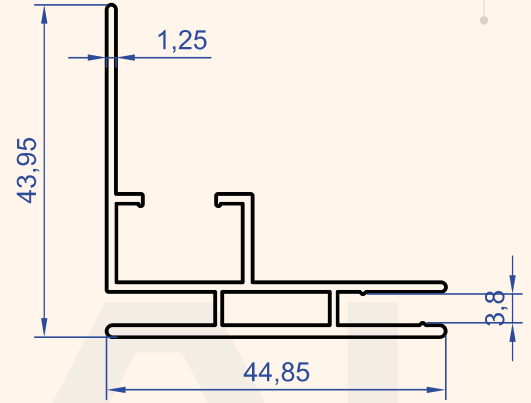
Profil No : 1151 Gramaj : 0.560 kg/m
