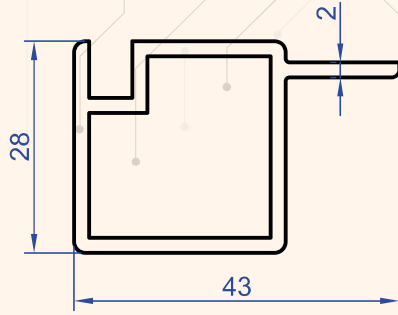
Profil No : 7239 Gramaj : 0.679 kg/m
