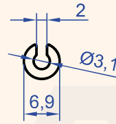
Profil No : 1093 Gramaj : 0.842 kg/m
