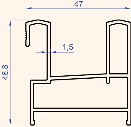
Profil No : 1094 Gramaj : 0.929 kg/m
