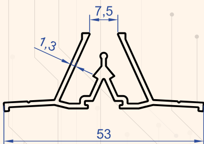
Profil No : 1380 Gramaj : 0.414 kg/m
