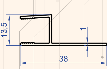
Profil No : 1229 Gramaj : 0.175 kg/m
