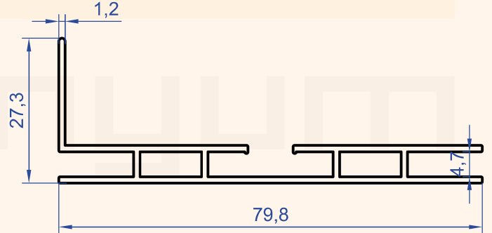
Profil No : 1150 Gramaj : 0.617 kg/m
