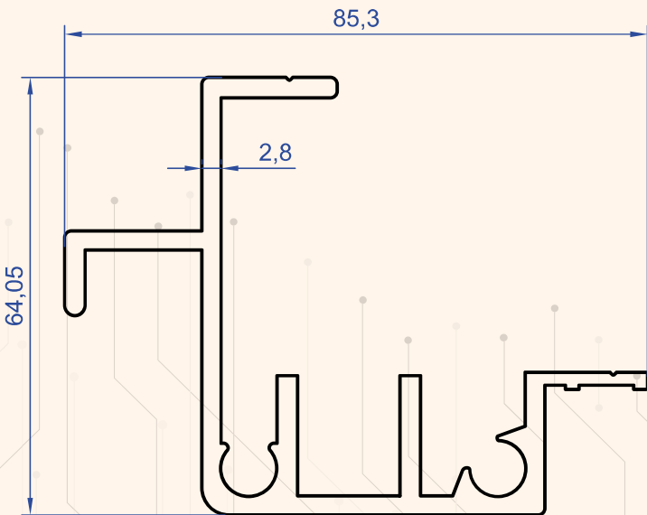
Profil No : 9209 Gramaj : 1.797 kg/m
