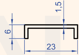
Profil No : 8990 Gramaj : 0.126 kg/m
