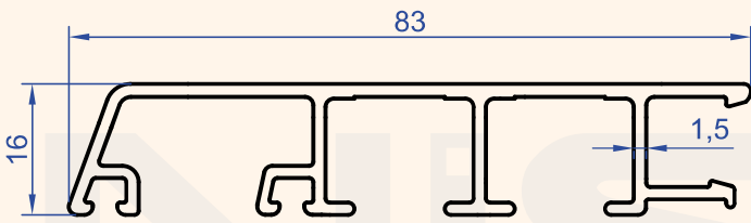
Profil No : 1081 Gramaj : 0.793 kg/m
