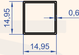
Profil No : 1368 Gramaj : 0.090 kg/m
