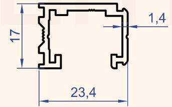
Profil No : 1161 Gramaj : 0.293 kg/m
