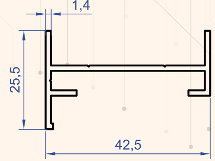
Profil No : 1142 Gramaj : 0.353 kg/m
