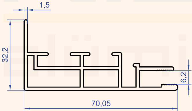
Profil No : 1353 Gramaj : 0.915 kg/m
