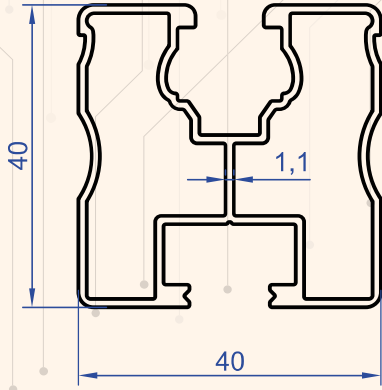
Profil No : 1398 Gramaj : 0.750 kg/m
