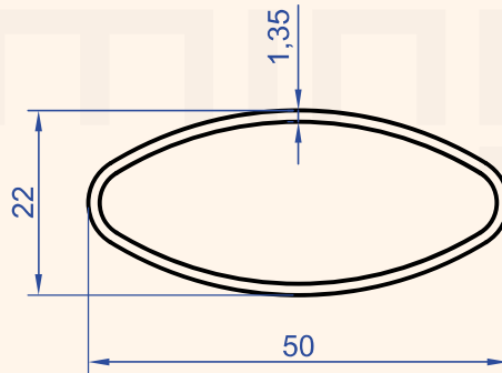
Profil No : 1269 Gramaj : 0.411 kg/m
