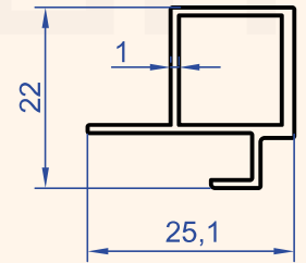
Profil No : 7240 Gramaj : 0.236 kg/m
