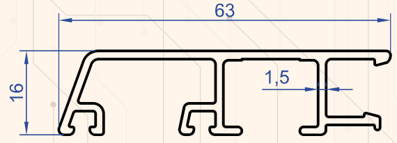
Profil No : 1082 Gramaj : 0.613 kg/m
