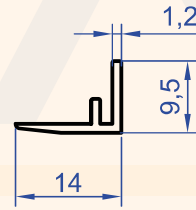
Profil No : 1393 Gramaj : 0.077 kg/m
