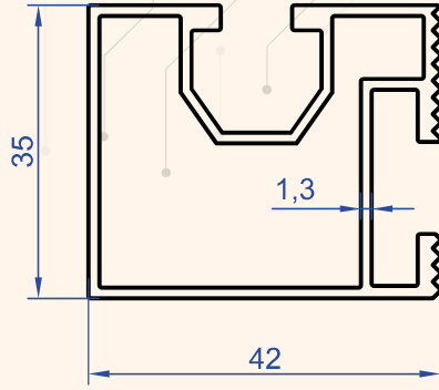
Profil No : 1394 Gramaj : 0.780 kg/m
