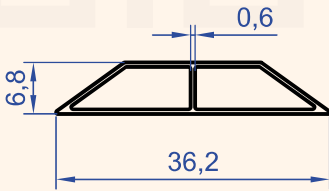
Profil No : 1002 Gramaj : 0.140 kg/m
