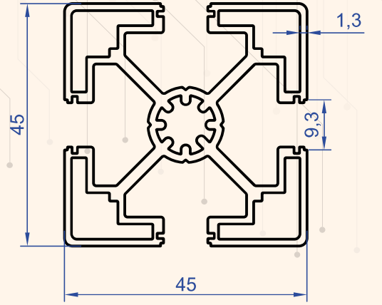
Profil No : 1382 Gramaj : 1.443 kg/m
