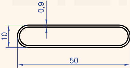
Profil No : 1084 Gramaj : 0.264 kg/m
