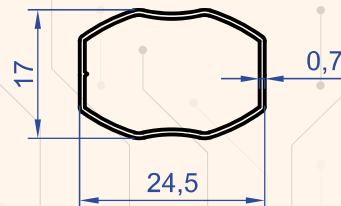
Profil No : 1153 Gramaj : 0.131 kg/m
