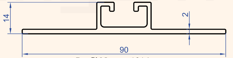
Profil No : 1214 Gramaj : 0.738 kg/m
