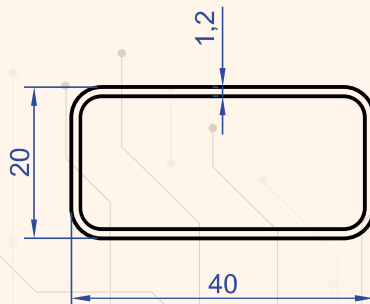
Profil No : 4824 Gramaj : 0.350 kg/m
