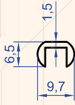
Profil No : 1241 Gramaj : 0.073 kg/m
