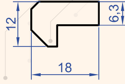
Profil No : 1362 Gramaj : 0.381 kg/m
