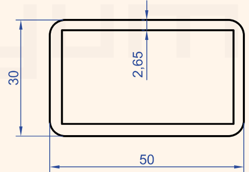
Profil No : 1170 Gramaj : 1.128 kg/m
