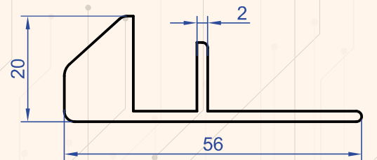
Profil No : 1199 Gramaj : 0.854 kg/m
