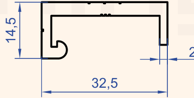
Profil No : 1160 Gramaj : 0.457 kg/m
