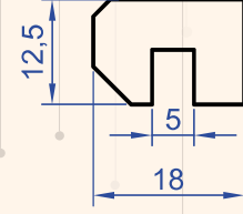
Profil No : 1363 Gramaj : 0.488 kg/m
