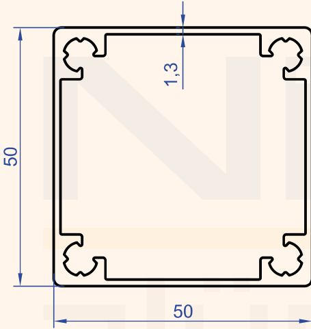
Profil No : 1141 Gramaj : 1.013 kg/m
