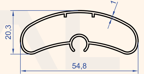
Profil No : 1076 Gramaj : 0.385 kg/m
