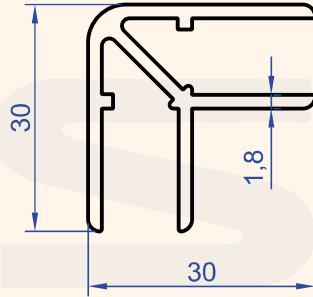
Profil No : 1340 Gramaj : 0.528 kg/m
