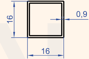
Profil No : 1030 Gramaj : 0.143 kg/m
