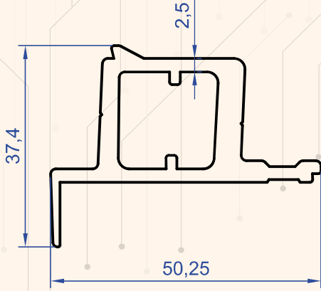
Profil No : 1158 Gramaj : 1.072 kg/m
