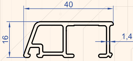
Profil No : 1083 Gramaj : 0.443 kg/m
