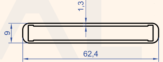
Profil No : 1193 Gramaj : 0.500 kg/m
