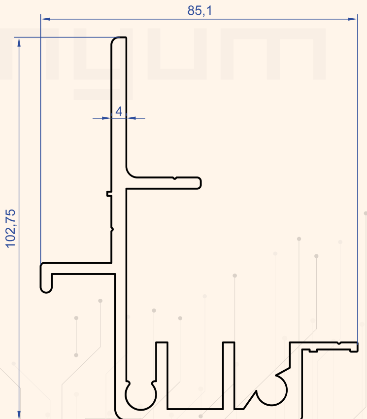
Profil No : 9208 Gramaj : 2.405 kg/m
