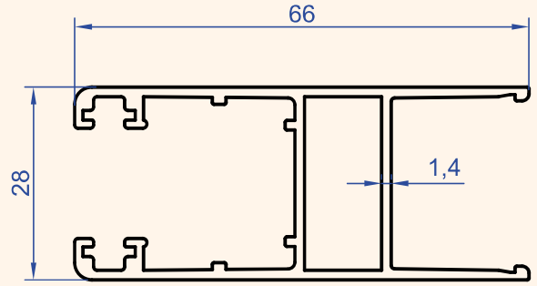
Profil No : 1093 Gramaj : 0.842 kg/m
