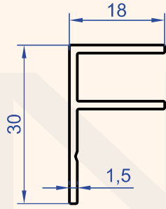
Profil No : 1339 Gramaj : 0.255 kg/m
