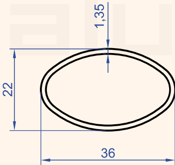
Profil No : 1268 Gramaj : 0.319 kg/m
