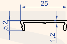
Profil No : 7193 Gramaj : 0.111 kg/m
