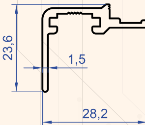
Profil No : 1162 Gramaj : 0.276 kg/m
