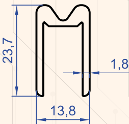
Profil No : 1337 Gramaj : 0.323 kg/m
