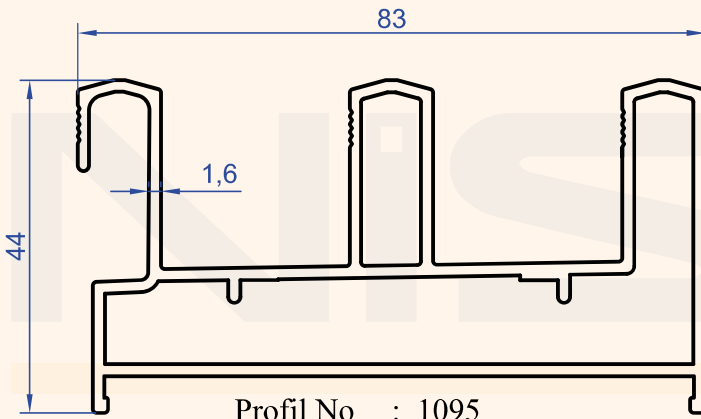
Profil No : 1095 Gramaj : 1.480 kg/m
