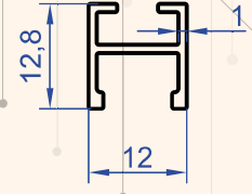
Profil No : 1180 Gramaj : 0.118 kg/m
