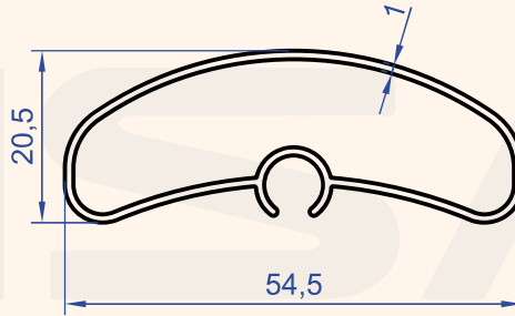
Profil No : 1114 Gramaj : 0.378 kg/m
