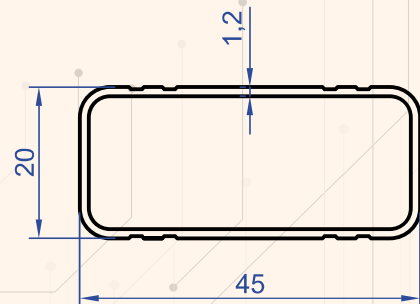
Profil No : 7966 Gramaj : 0.376 kg/m
