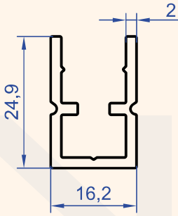
Profil No : 1184 Gramaj : 0.363 kg/m
