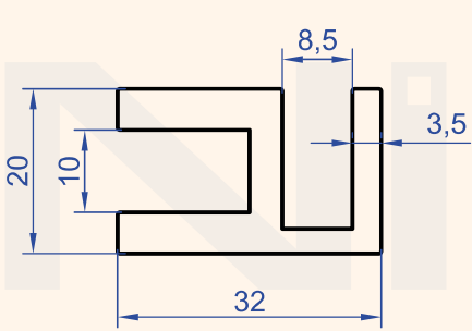
Profil No : 1052 Gramaj : 0.908 kg/m
