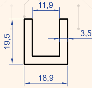
Profil No : 1378 Gramaj : 0.482 kg/m
