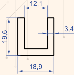
Profil No : 1272 Gramaj : 0.472 kg/m
