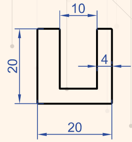
Profil No : 1051 Gramaj : 0.650 kg/m
