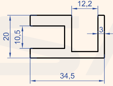
Profil No : 1397 Gramaj : 0.852 kg/m
