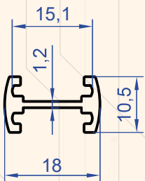
Profil No : 1156 Gramaj : 0.166 kg/m
