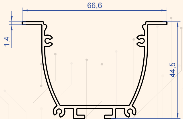
Profil No : 1163 Gramaj : 0.679 kg/m
