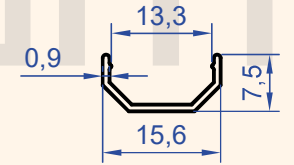
Profil No : 1207 Gramaj : 0.061 kg/m
