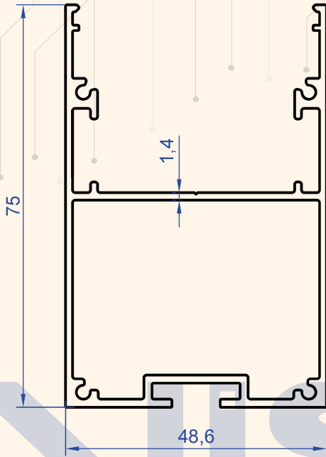
Profil No : 1275 Gramaj : 1.130 kg/m
