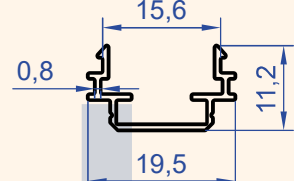
Profil No : 1205 Gramaj : 0.103 kg/m
