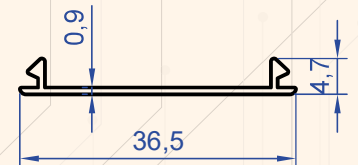
Profil No : 9823 Gramaj : 0.116 kg/m
