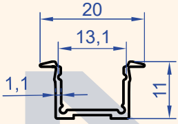
Profil No : 1110 Gramaj : 0.106 kg/m
