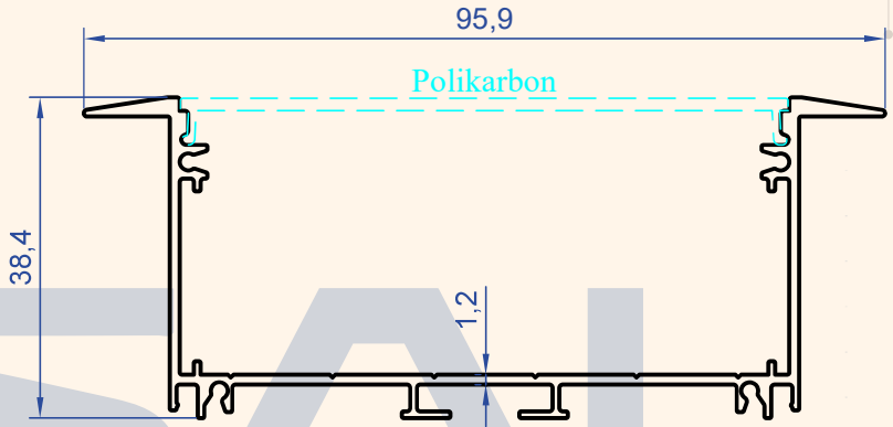
Profil No : 1312 Gramaj : 0.704 kg/m
