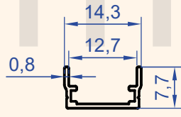
Profil No : 1301 Gramaj : 0.067 kg/m
