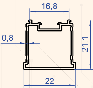
Profil No : 1011 Gramaj : 0.198 kg/m
