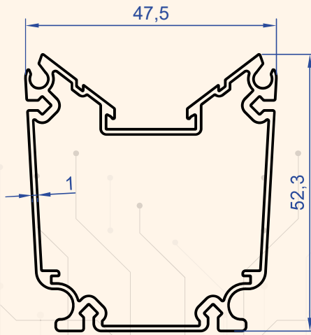
Profil No : 1216 Gramaj : 0.821 kg/m
