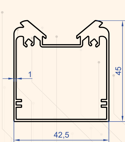
Profil No : 1240 Gramaj : 0.829 kg/m
