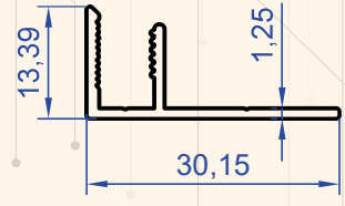
Profil No : 1361 Gramaj : 0.184 kg/m
