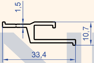
Profil No : 1273 Gramaj : 0.238 kg/m
