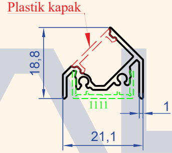
Profil No : 1360 Gramaj : 0.304 kg/m
