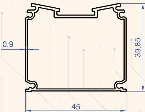
Profil No : 1182 Gramaj : 0.512 kg/m
