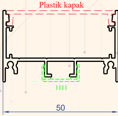
Profil No : 1396 Gramaj : 0.563 kg/m
