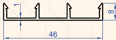
Profil No : 1321 Gramaj : 0.227 kg/m
