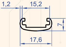
Profil No : 1228 Gramaj : 0.122 kg/m
