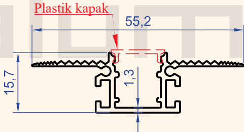
Profil No : 1358 Gramaj : 0.360 kg/m
