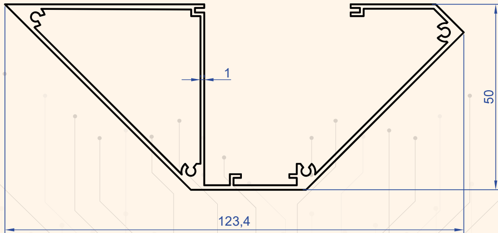
Profil No : 1243 Gramaj : 1.132 kg/m
