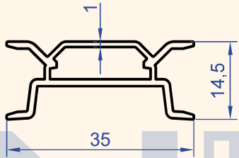
Profil No : 1043 Gramaj : 0.298 kg/m
