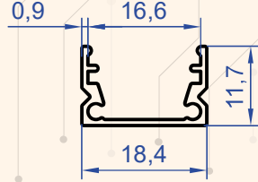
Profil No : 1252 Gramaj : 0.133 kg/m
