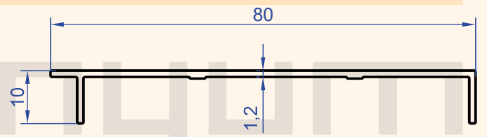
Profil No : 1299 Gramaj : 0.321 kg/m
