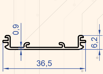
Profil No : 9824 Gramaj : 0.143 kg/m
