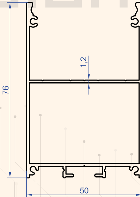
Profil No : 1264 Gramaj : 0.978 kg/m
