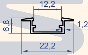
Profil No : 1389 Gramaj : 0.086 kg/m
