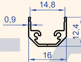
Profil No : 1112 Gramaj : 0.132 kg/m
