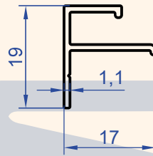
Profil No : 1367 Gramaj : 0.139 kg/m
