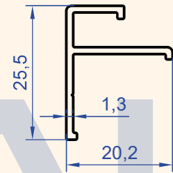
Profil No : 1274 Gramaj : 0.199 kg/m
