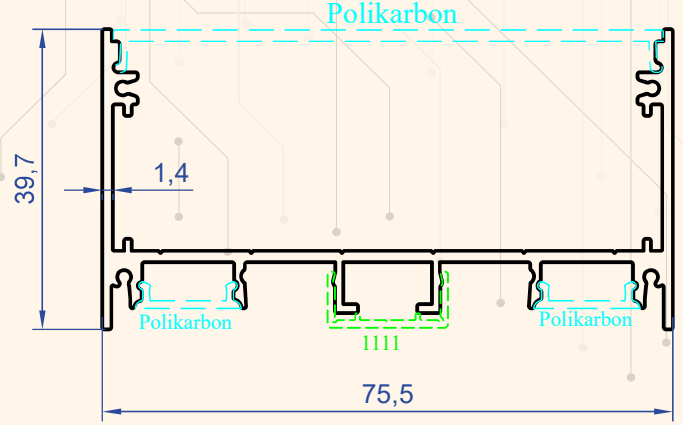
Profil No : 1313 Gramaj : 0.829 kg/m
