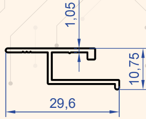
Profil No : 1016 Gramaj : 0.154 kg/m
