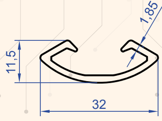
Profil No : 1374 Gramaj : 0.253 kg/m
