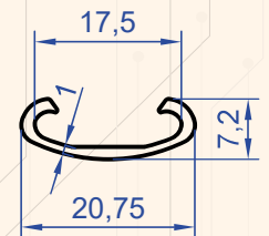
Profil No : 1286 Gramaj : 0.108 kg/m
