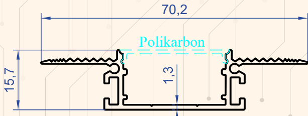
Profil No : 1344 Gramaj : 0.398 kg/m
