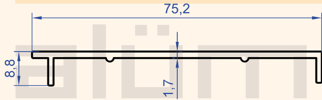
Profil No : 1107 Gramaj : 0.404 kg/m
