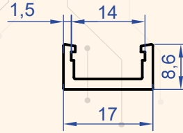
Profil No : 1102 Gramaj : 0.159 kg/m
