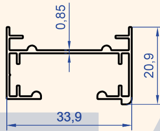
Profil No : 9746 Gramaj : 0.263 kg/m
