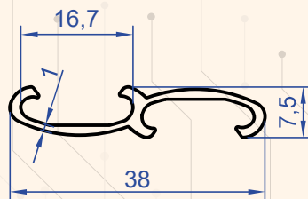
Profil No : 1157 Gramaj : 0.203 kg/m
