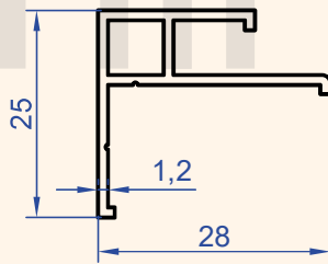
Profil No : 1351 Gramaj : 0.256 kg/m
