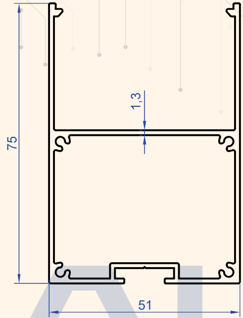
Profil No : 1078 Gramaj : 1.032 kg/m
