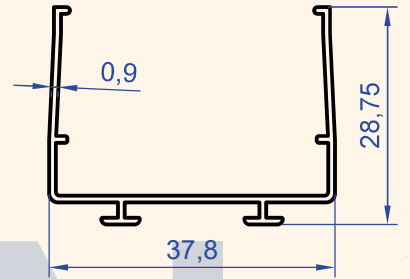
Profil No : 9822 Gramaj : 0.258 kg/m
