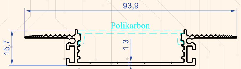
Profil No : 1371 Gramaj : 0.494 kg/m
