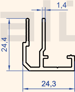
Profil No : 1293 Gramaj : 0.324 kg/m
