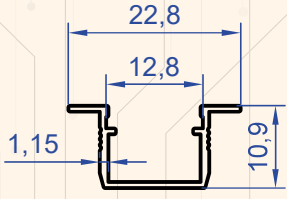
Profil No : 1251 Gramaj : 0.107 kg/m
