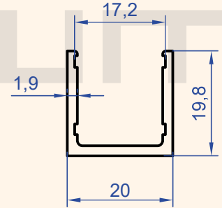
Profil No : 1198 Gramaj : 0.276 kg/m
