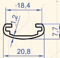
Profil No : 1377 Gramaj : 0.134 kg/m
