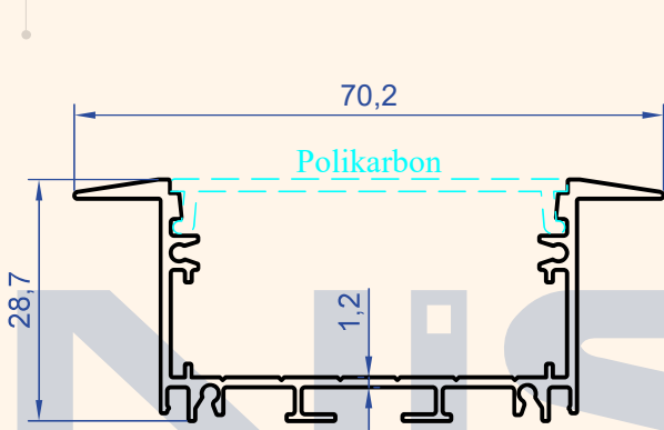
Profil No : 1311 Gramaj : 0.560 kg/m
