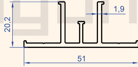
Profil No : 1395 Gramaj : 0.501 kg/m
