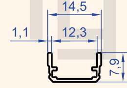
Profil No : 1206 Gramaj : 0.071 kg/m
