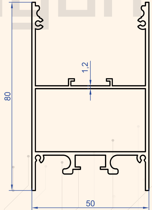
Profil No : 1270 Gramaj : 1.269 kg/m
