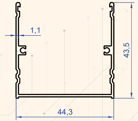
Profil No : 1155 Gramaj : 0.445 kg/m
