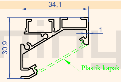
Profil No : 1359 Gramaj : 0.378 kg/m
