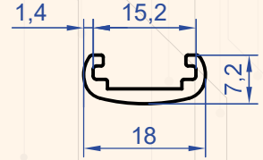
Profil No : 1101 Gramaj : 0.137 kg/m
