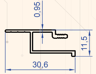
Profil No : 1023 Gramaj : 0.163 kg/m
