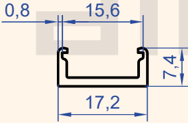
Profil No : 1245 Gramaj : 0.123 kg/m
