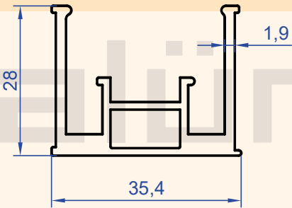
Profil No : 1325 Gramaj : 0.679 kg/m
