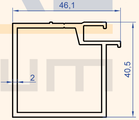
Profil No : 1317 Gramaj : 0.896 kg/m
